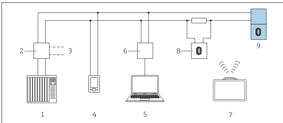
图 11 通过 HART 通信实现远程操作
