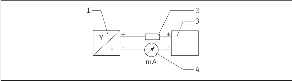
图 5 HART 信号回路连接框图
