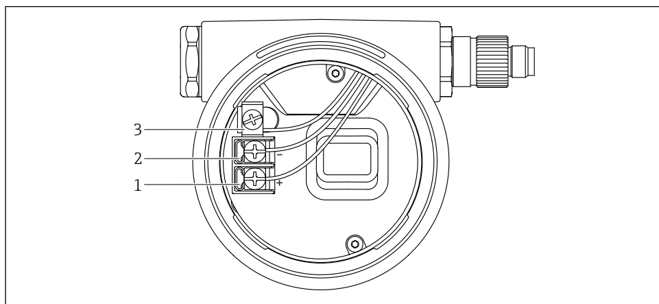
图 6 接线腔中的接线端子和接地端
