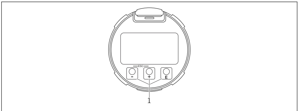
10 图形显示屏，带光敏按键 (1)
