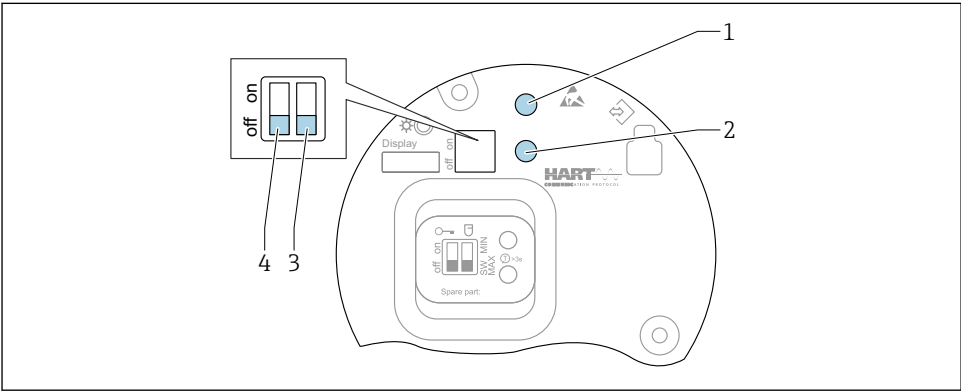
图 9 HART 电子插件上的操作按键和 DIP 开关
