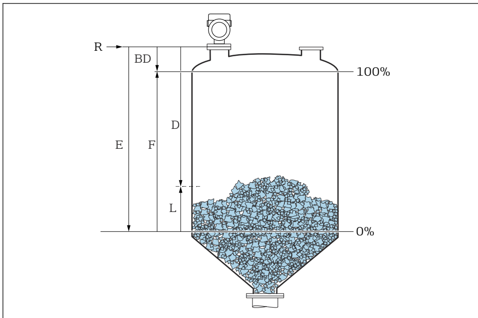
图 12 料位测量设置参数
