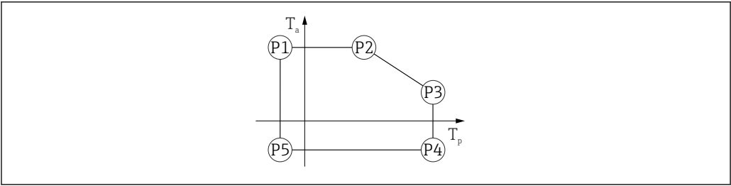
图 17 塑料外壳材质；过程温度范围：-20 ... +150 °C (-4 ... +302 °F)
