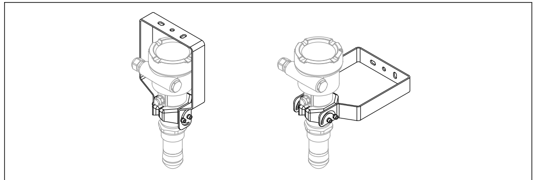
图 15 安装在罐顶或墙壁上
