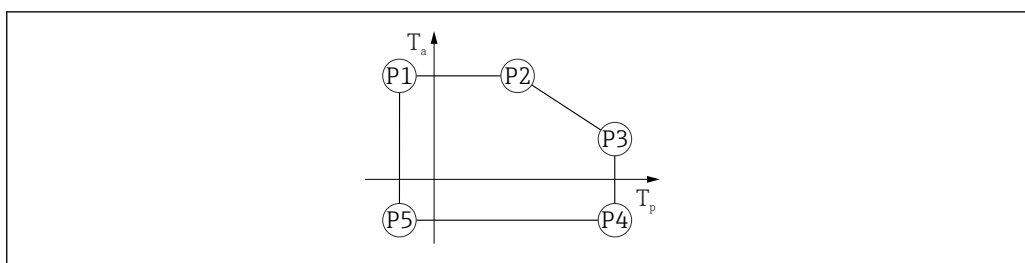
25 塑料外壳材质; 过程温度范围: -40 \dots +150^\circ\text{C} ( -40 \dots +302^\circ\text{F} )
