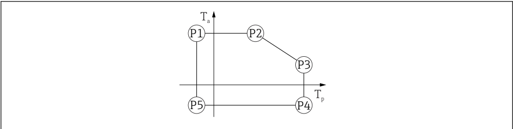
35 316L 外壳材质；过程温度范围：-20 ... +150 °C (-4 ... +302 °F)
