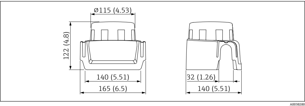
图 14 外形尺寸示意图。测量单位 mm (in)
