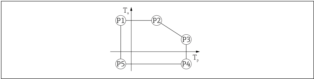
图 39 316L 外壳材质；过程温度范围：-40 ... +200 °C (-40 ... +392 °F)
