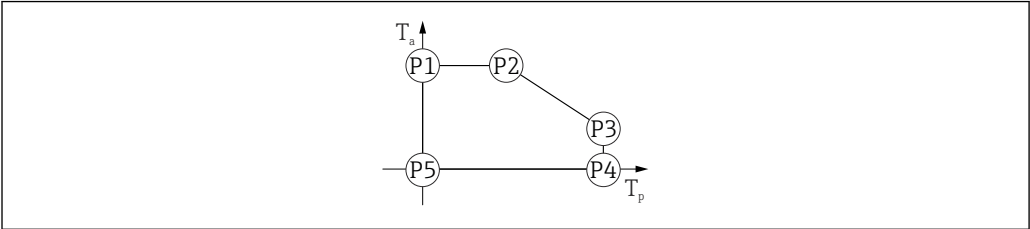
图 28 塑料外壳材质；过程温度范围：0 ... +200 °C (+32 ... +392 °F)，适用 CSA C/US 认证型仪表
