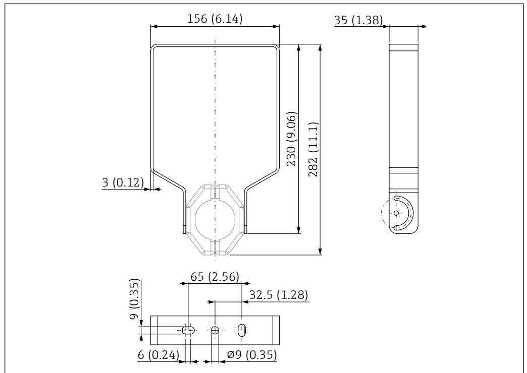
图 16 安装架的外形尺寸示意图。测量单位 mm (in)
