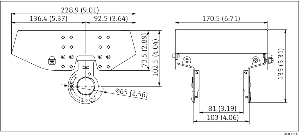
图 13 外形尺寸示意图。测量单位 mm (in)
