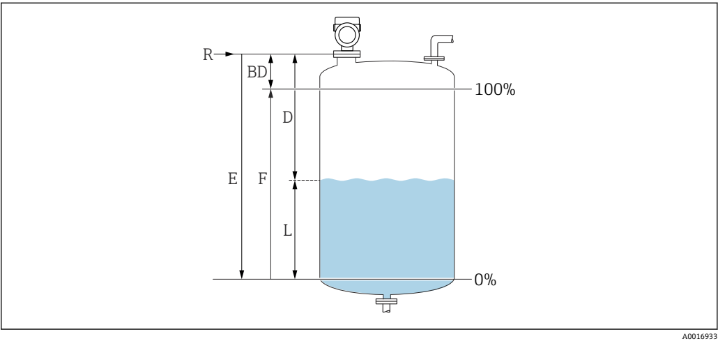
图 10 液位测量的设置参数
