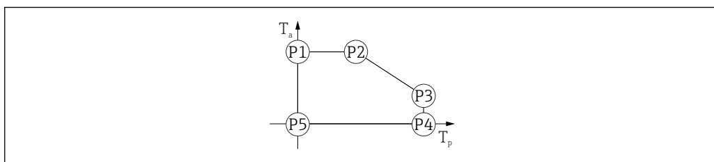
20 塑料外壳材质; 过程温度范围: 0 \dots +150\text{ }^{\circ}\text{C} ( +32 \dots +302\text{ }^{\circ}\text{F} ), 适用 CSA C/US 认证型仪表
