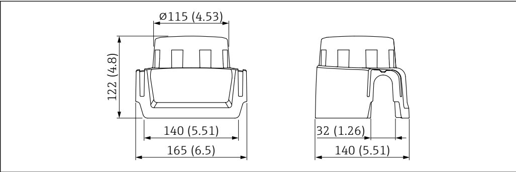
图 14 外形尺寸示意图。测量单位 mm (in)
