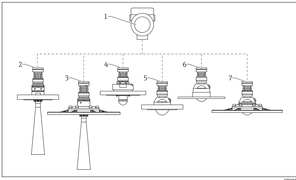
图 1 Micropilot FMR67B 的结构设计
