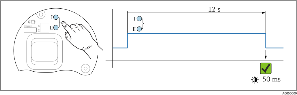
图 15 电子插件上的操作按键
