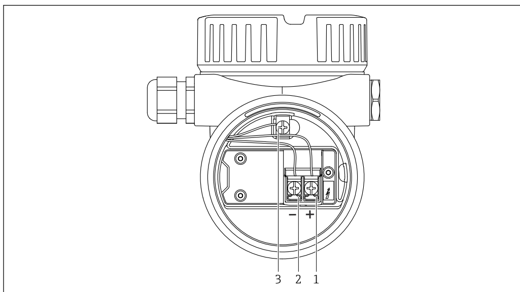
图 9 接线腔中的接线端子和接地端
