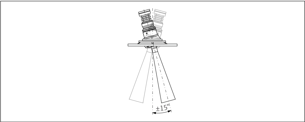
2 喇叭天线，带天线角度调节装置
