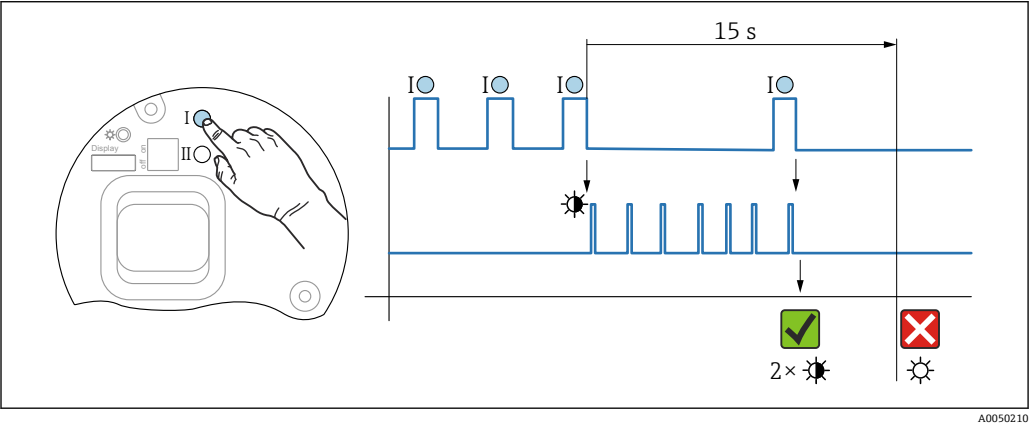
图 14 操作步骤 - 重置密码
