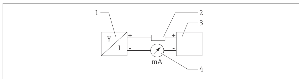
图 6 HART 信号回路连接框图
