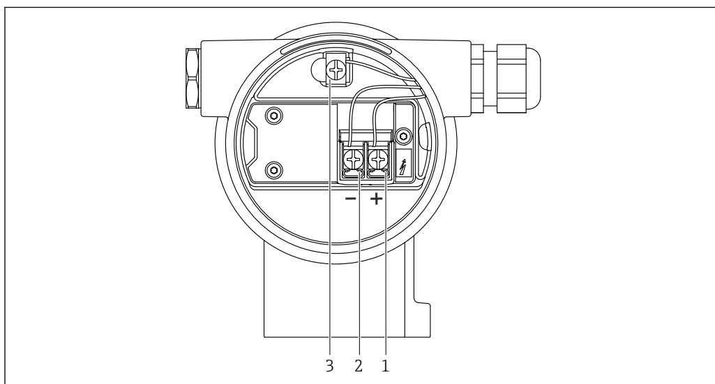
图 8 接线腔中的接线端子和接地端
