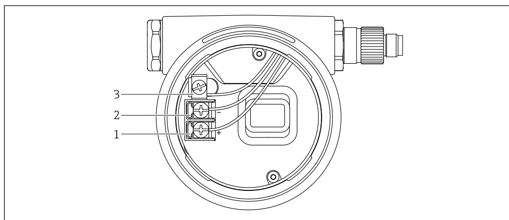
图 7 接线腔中的接线端子和接地端
