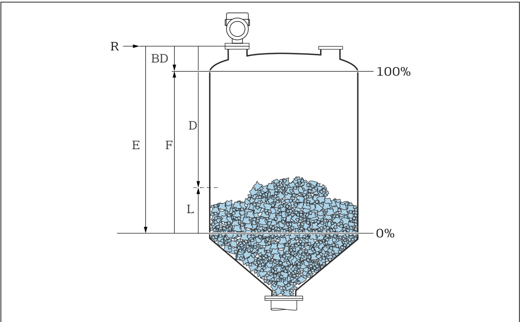
图 13 料位测量设置参数
