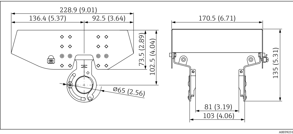
图 16 外形尺寸示意图。测量单位 mm (in)
