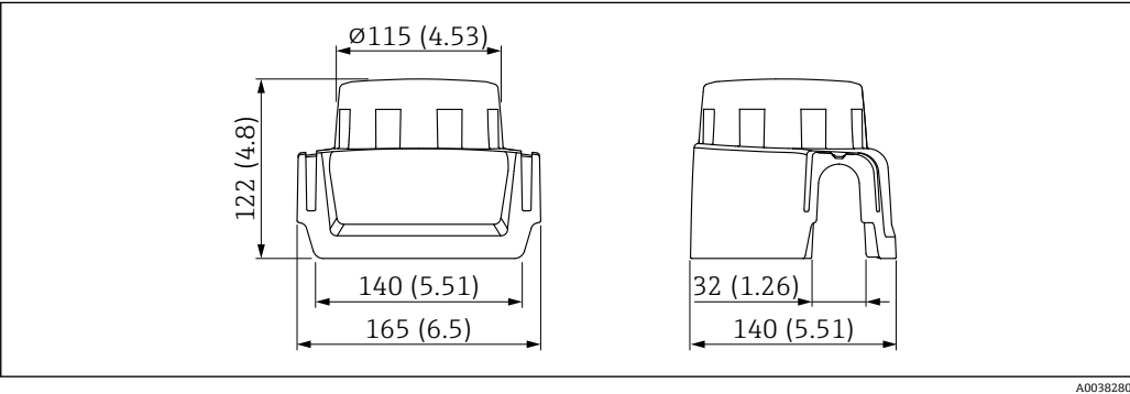
图 17 外形尺寸示意图。测量单位 mm (in)
