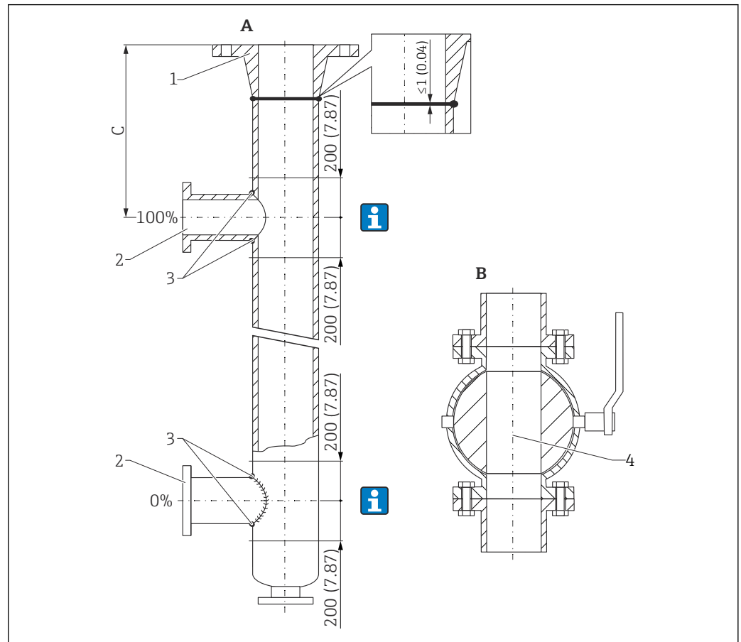
图 11 旁通管设计实例。测量单位 mm (in)
