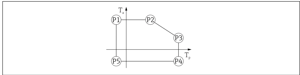
图 34 铝外壳材质；过程温度范围：-60 ... +150 °C (-76 ... +302 °F)
