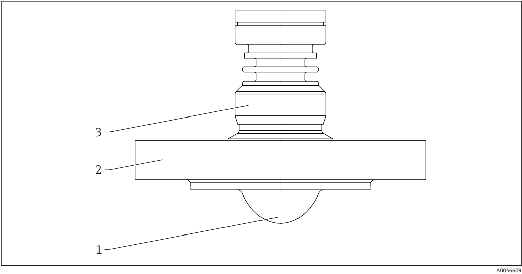
图 54 PTFE 涂层天线（齐平安装，50 mm (2 in)口径）的材质；带法兰
