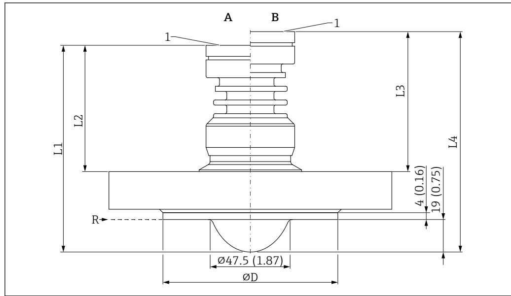
图 50 PTFE 涂层天线（齐平安装，50 mm (2 in)口径）的外形尺寸示意图；带法兰。测量单位 mm (in)
