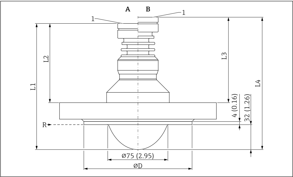
51 PTFE 涂层天线（齐平安装，80 mm (3 in)口径）的外形尺寸示意图；带法兰。测量单位 mm (in) A 过程温度 ≤ 150 °C (302 °F)的仪表型号 B 过程温度 ≤ 200 °C (392 °F)的仪表型号 R 测量参考点 1 外壳底部 ØD 涂层 = 密封面，符合 ASME B16.5 / EN1092-1 / JIS B2220 法兰标准 L1 157 mm (6.18 in); Ex d/XP 防爆认证型仪表: +5 mm (+0.20 in) L2 尺寸因法兰厚度而异 (标准法兰) L3 尺寸因法兰厚度而异 (标准法兰) L4 169 mm (6.65 in); Ex d/XP 防爆认证型仪表: +5 mm (+0.20 in)
