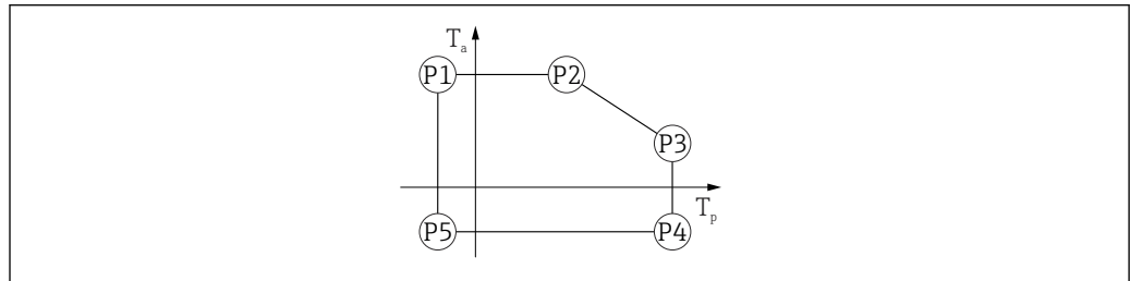
图 22 塑料外壳材质；过程温度范围：-40 ... +450 °C (-40 ... +842 °F)
