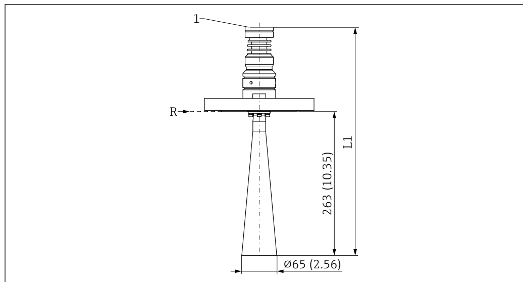
图 48 DN65 喇叭天线的外形尺寸示意图; 法兰过程连接。测量单位 mm (in)
