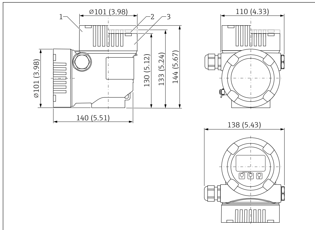
图 47 双腔室外壳 (L 型) 的外形尺寸示意图
