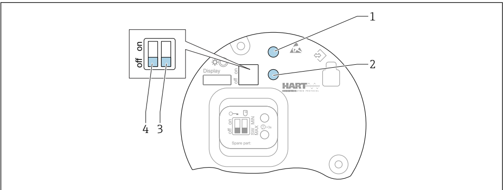
图 56 HART 电子插件上的操作按键和 DIP 开关
