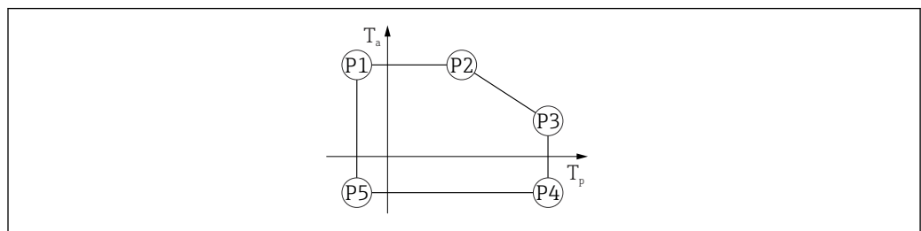
29 铝外壳材质；过程温度范围：-20 ... +200 °C (-4 ... +392 °F)
