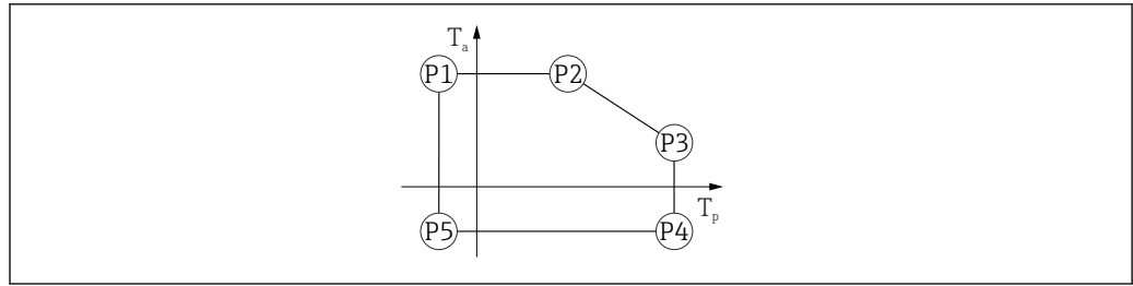
图 33 铝外壳材质；过程温度范围：-40 ... +450 °C (-40 ... +842 °F)
