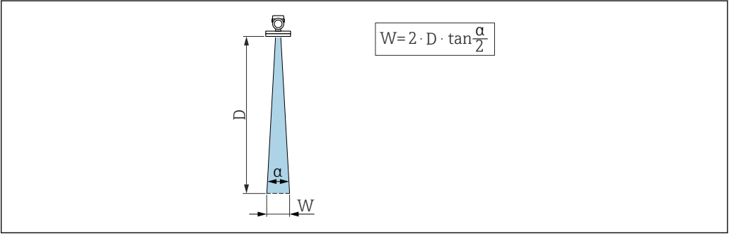
7 波束角 \alpha 、距离 D 和波束宽度 W 的相互关系
