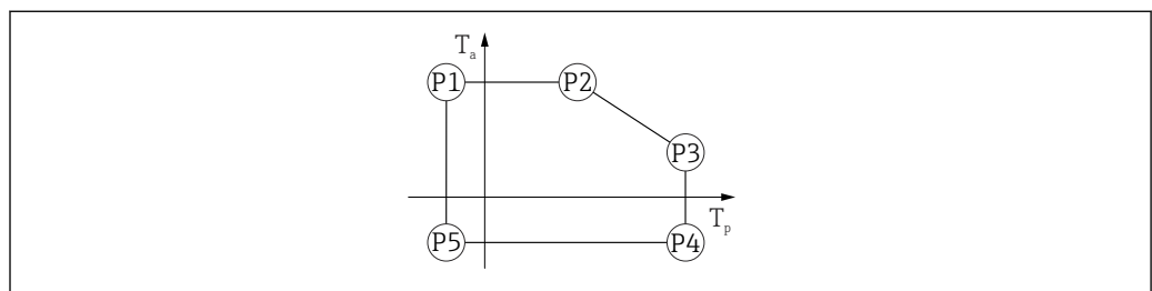
41 316L 外壳材质; 过程温度范围: -40 \dots +450 \text{ }^{\circ}\text{C} ( -40 \dots +842 \text{ }^{\circ}\text{F} )
