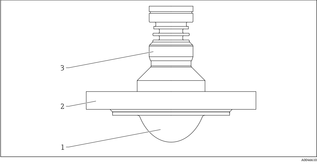
图 55 PTFE 涂层天线（齐平安装，80 mm (3 in)口径）的材质；带法兰
