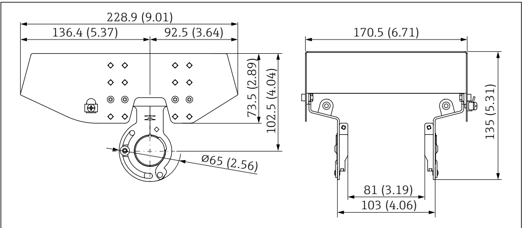
图 58 外形尺寸示意图。测量单位 mm (in)
