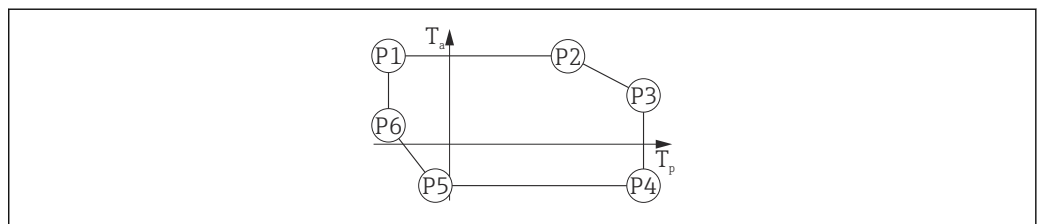
26 单腔室塑料外壳；过程温度范围：-196 ... +200 °C (-320 ... +392 °F)
