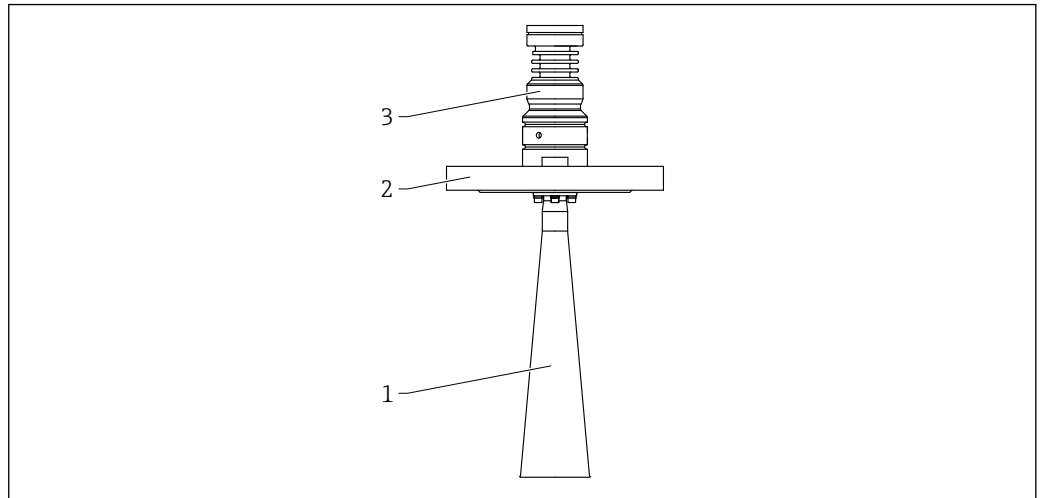
■ 52 DN65 喇叭天线的材质。测量单位 mm (in)
