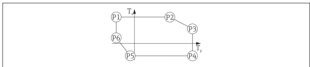
图 35 铝外壳材质；过程温度范围：-196 ... +200 °C (-320 ... +392 °F)
