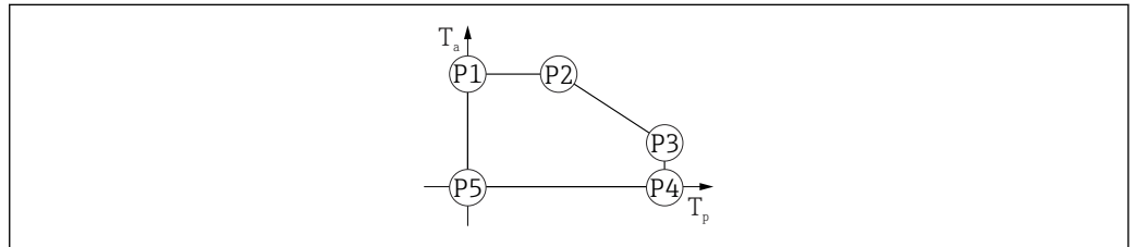
25 塑料外壳材质；过程温度范围：0 ... +150 °C (+32 ... +302 °F)，适用 CSA C/US 认证型仪表
