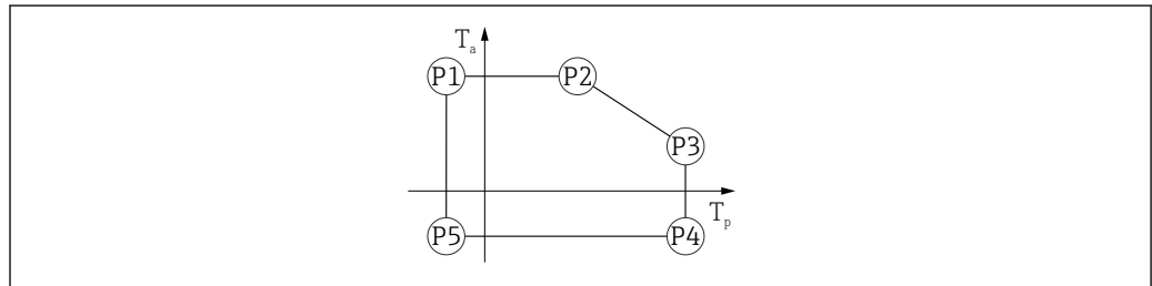
40 316L 外壳材质; 过程温度范围: -40 \dots +280 \text{ }^{\circ}\text{C} ( -40 \dots +536 \text{ }^{\circ}\text{F} )
