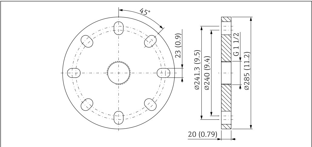
图 28 UNI 6"/DN150/150A 法兰的外形尺寸示意图。测量单位 mm (in)
