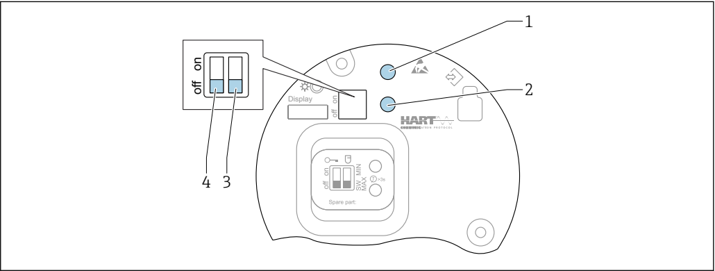
图 31 HART 电子插件上的操作按键和 DIP 开关
