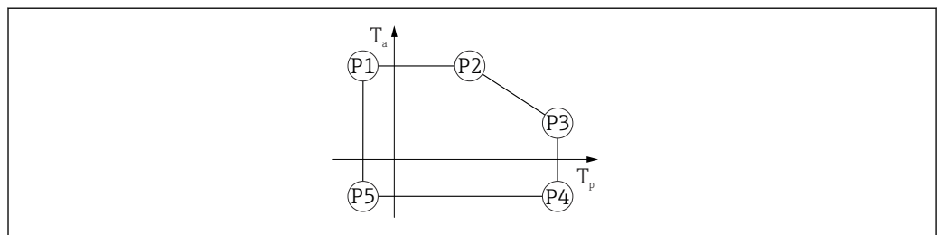
10 塑料外壳材质；过程温度范围：-40 ... +130 °C (-40 ... +266 °F)
