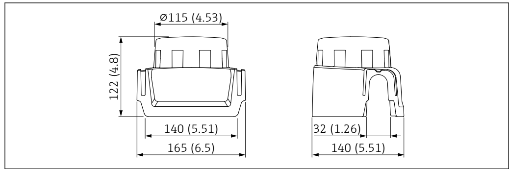
图 34 外形尺寸示意图。测量单位 mm (in)
