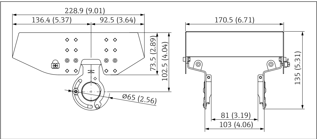
图 33 外形尺寸示意图。测量单位 mm (in)
