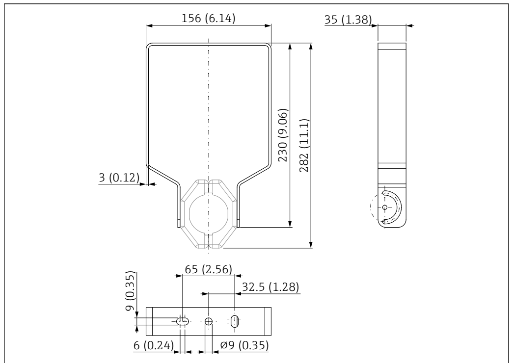
36 安装架的外形尺寸示意图。测量单位 mm (in)
