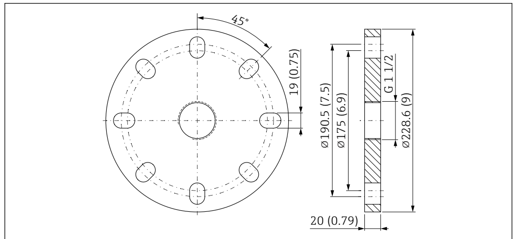
图 27 UNI 4"/DN100/100A 法兰的外形尺寸示意图。测量单位 mm (in)
