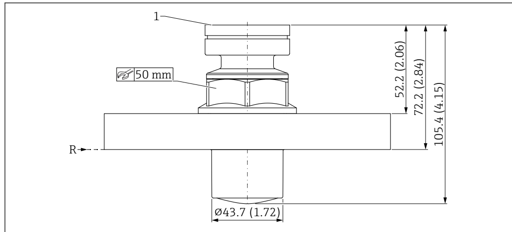
图 20 PVDF 全密封天线（40 mm (1.5 in) 口径）的外形尺寸示意图；UNI 法兰过程连接。测量单位 mm (in)
