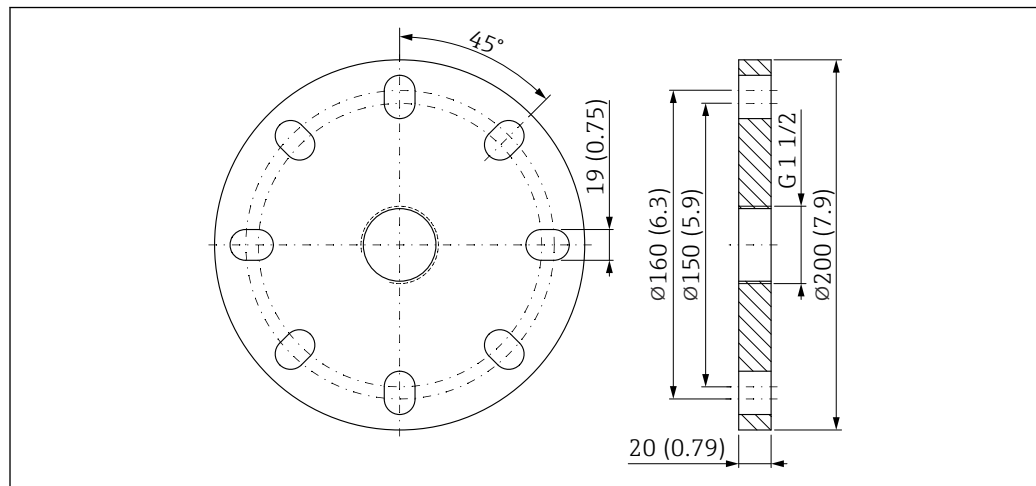
图 21 UNI 3"/DN80/80A 法兰的外形尺寸示意图。测量单位 mm (in)
