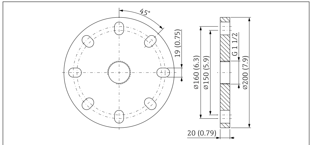
图 26 UNI 3"/DN80/80A 法兰的外形尺寸示意图。测量单位 mm (in)
