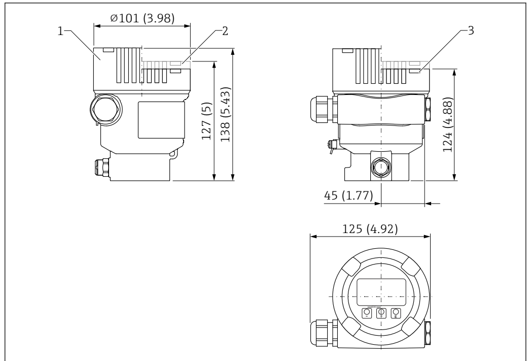
图 16 单腔室铝外壳的外形尺寸示意图
