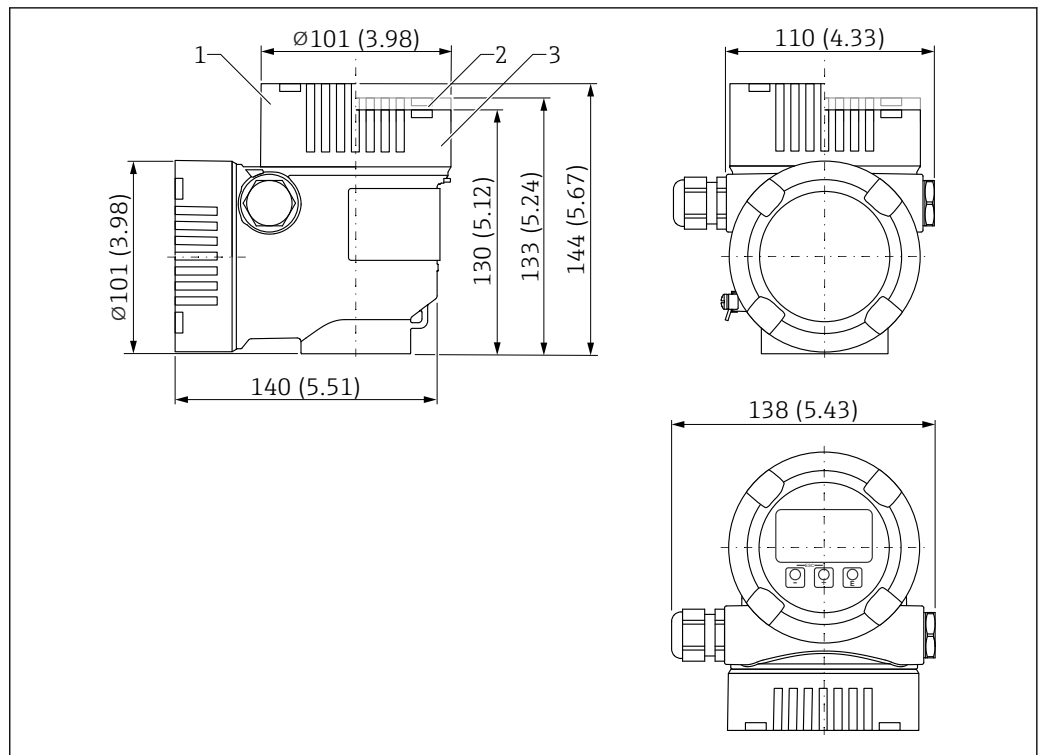
图 18 双腔室外壳 (L 型) 的外形尺寸示意图
