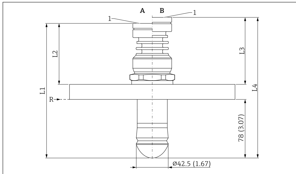
图 25 水滴型天线 (50 mm (2 in)口径) 的外形尺寸示意图；UNI 法兰过程连接。测量单位 mm (in)
