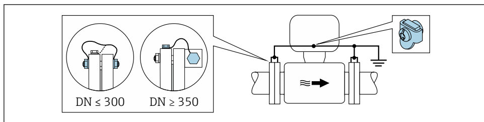
5 Compensation de potentiel via la borne de terre et les brides du tube
