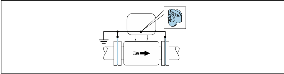
6 Compensation de potentiel via la borne de terre et les disques de mise à la terre ( PE = P_{FL} = P_M )
