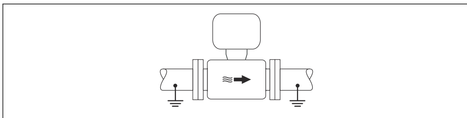
4 Compensation de potentiel via le tube de mesure
