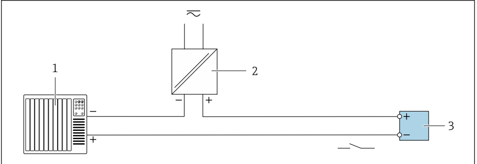
图 5 开关量输出(无源信号)的连接实例
