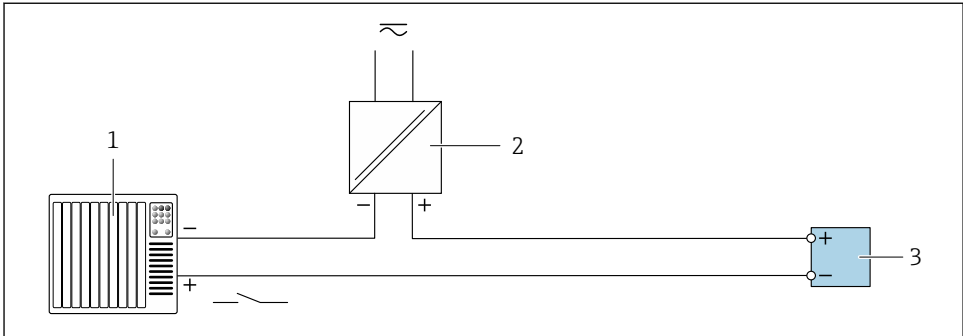
图 6 状态输入的连接示例
