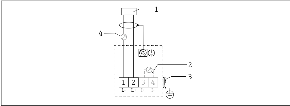
7 2선식 버전의 단자 할당
