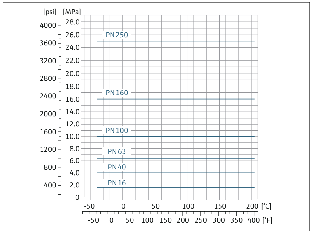
図 26 フランジ材質：ステンレス 1.4410/F53 25Cr 二相（スーパー二相）
