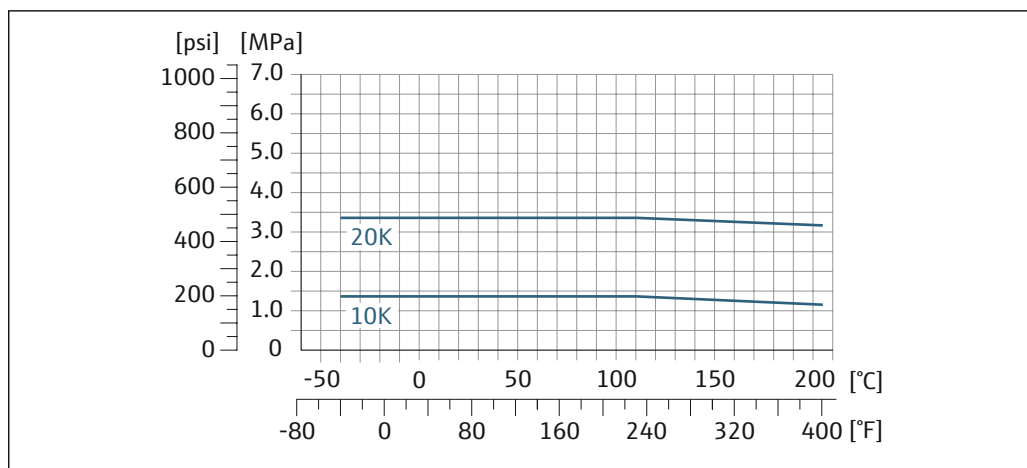
図 28 フランジ材質：ステンレス 1.4410/F53 25Cr 二相（スーパー二相）
