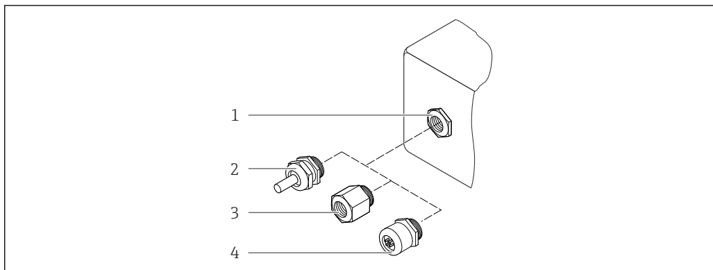
図 39 可能な電線管接続口/ケーブルグランド
