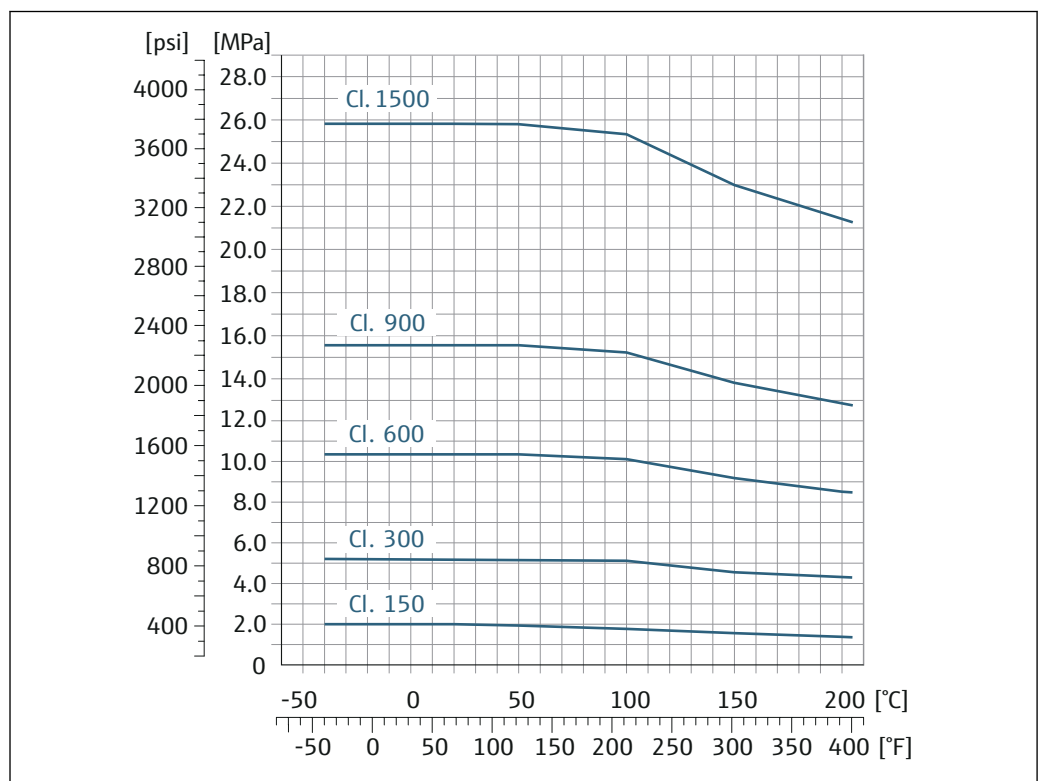
図 27 フランジ材質：ステンレス 1.4410/F53 25Cr 二相（スーパー二相）
