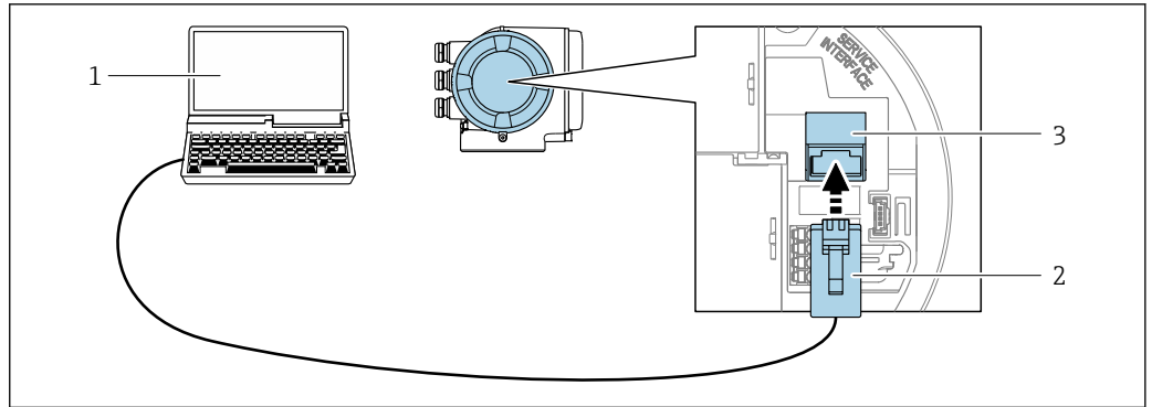
図 53 サービスインターフェイス (CDI-RJ45) 経由の接続
