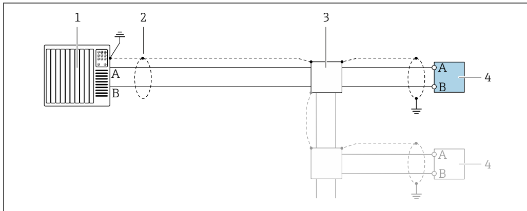
17 Пример подключения для интерфейса Modbus RS485, в невзрывоопасной зоне или зоне 2/разд. 2
