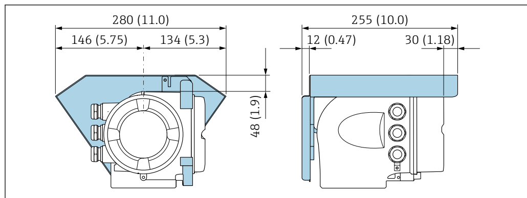
8 Защитный козырек от погодных явлений для прибора Proline 500; единицы измерения – мм (дюймы)
