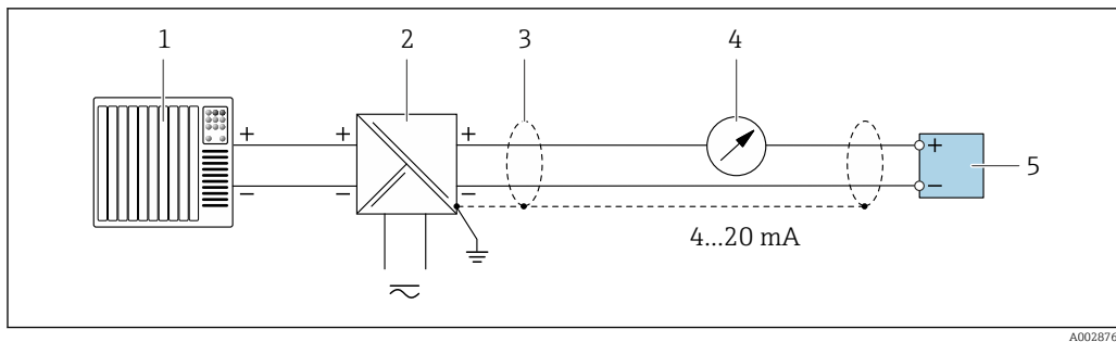
19 Пример подключения для токового выхода 4–20 мА HART (пассивного)
