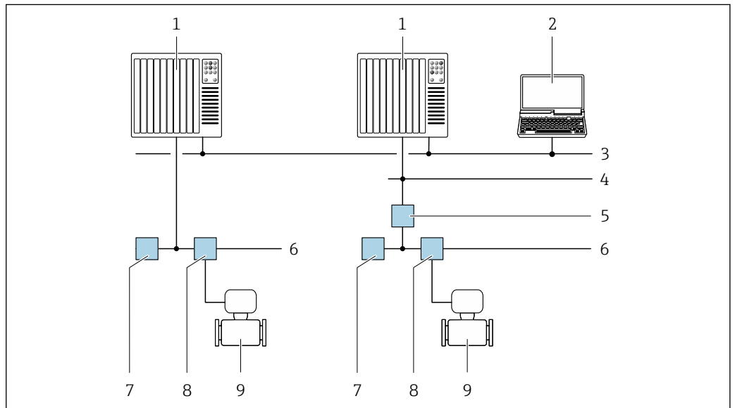
48 Варианты дистанционного управления через сеть FOUNDATION Fieldbus
