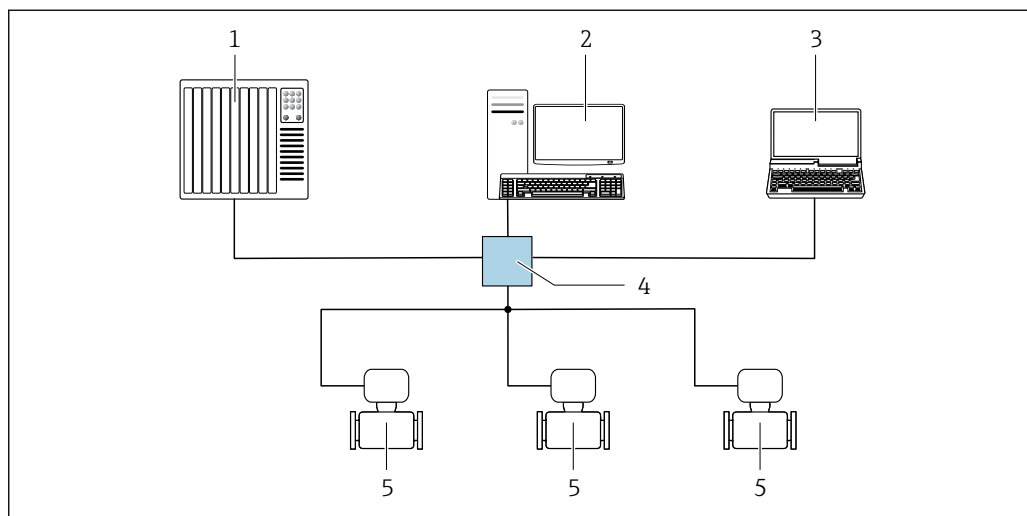
52 Варианты дистанционного управления через сеть EtherNet/IP: топология «звезда»
