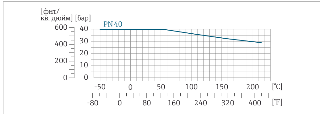
27 Поворотно-фланцевое соединение с фланцем из материала 1.4301 (F304), смачиваемые компоненты из сплава Alloy C22: 2.4602 (UNS N06022)
