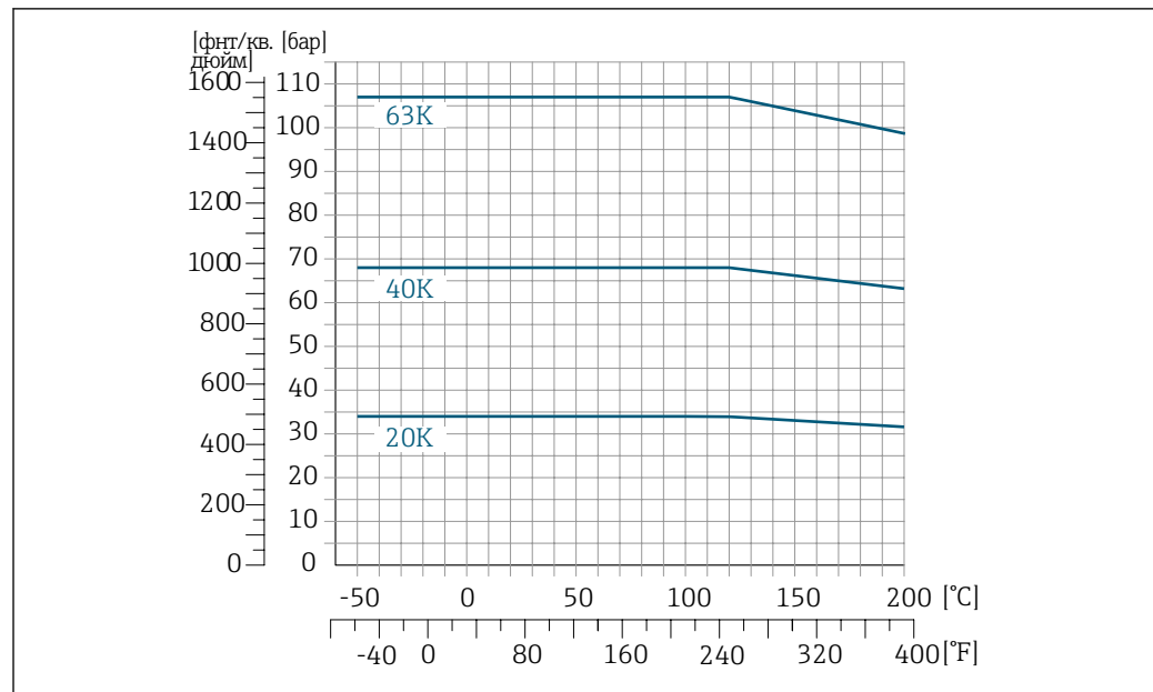
31 С фланцем из материала 1.4404 (316/316L) или сплава Alloy C22, 2.4602 (UNS N06022)
