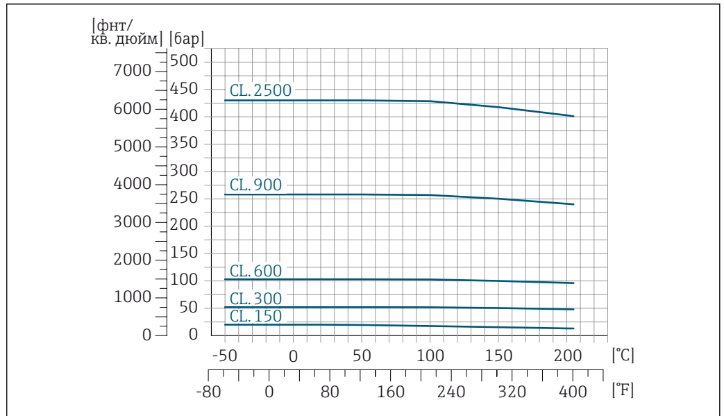
29 С фланцем из сплава Alloy C22, 2.4602 (UNS N06022)
