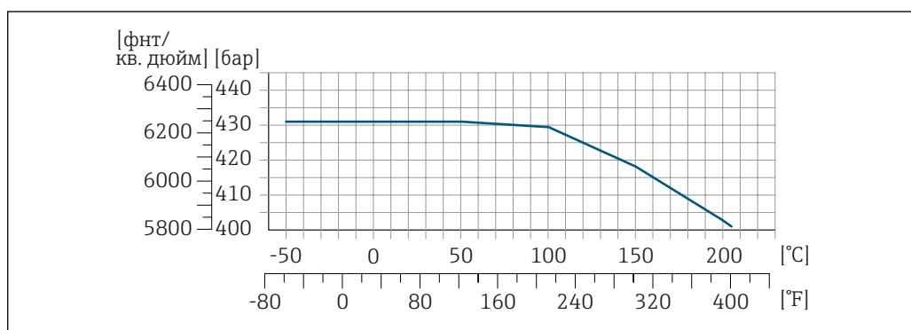
35 С фланцем из сплава Alloy C22, 2.4602 (UNS N06022); код заказа «Материал измерительной трубки, смачиваемая поверхность», опция HB
