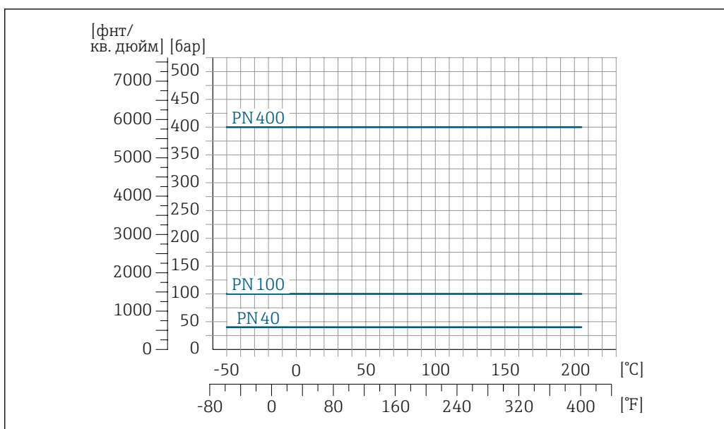
26 С фланцем из сплава Alloy C22, 2.4602 (UNS N06022)
