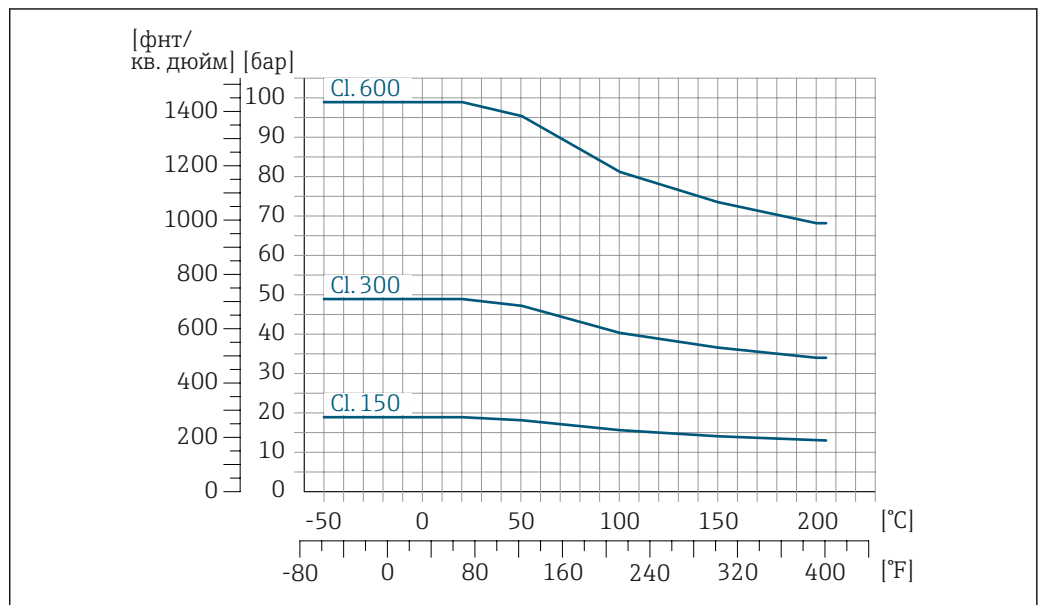
30 Поворотно-фланцевое соединение с фланцем из материала 1.4301 (F304), смачиваемые компоненты из сплава Alloy C22: 2.4602 (UNS N06022)
