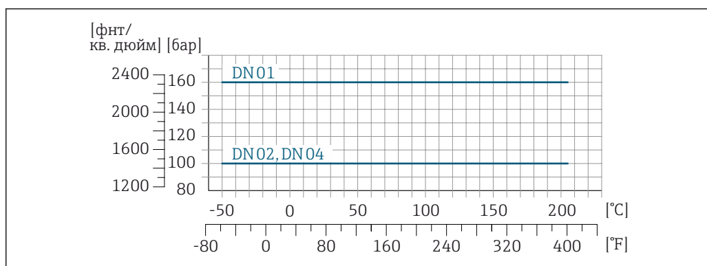
33 С фланцем из материала 1.4404 (316/316L)
