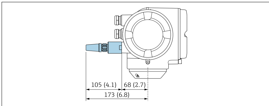
43 Единицы измерения – мм (дюймы)
