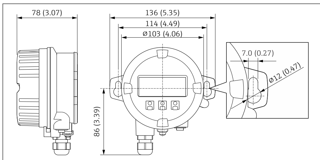
42 Единица измерения – мм (дюймы)
