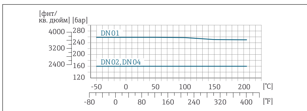
34 С фланцем из сплава Alloy C22, 2.4602 (UNS N06022)
