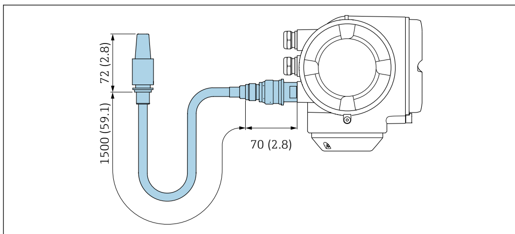
44 Единицы измерения – мм (дюймы)
