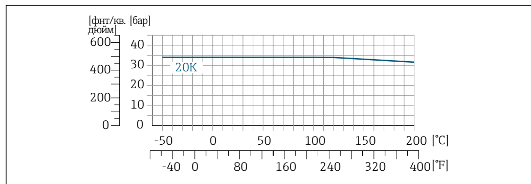
32 Поворотно-фланцевое соединение с фланцем из материала 1.4301 (F304), смачиваемые компоненты из сплава Alloy C22: 2.4602 (UNS N06022)
