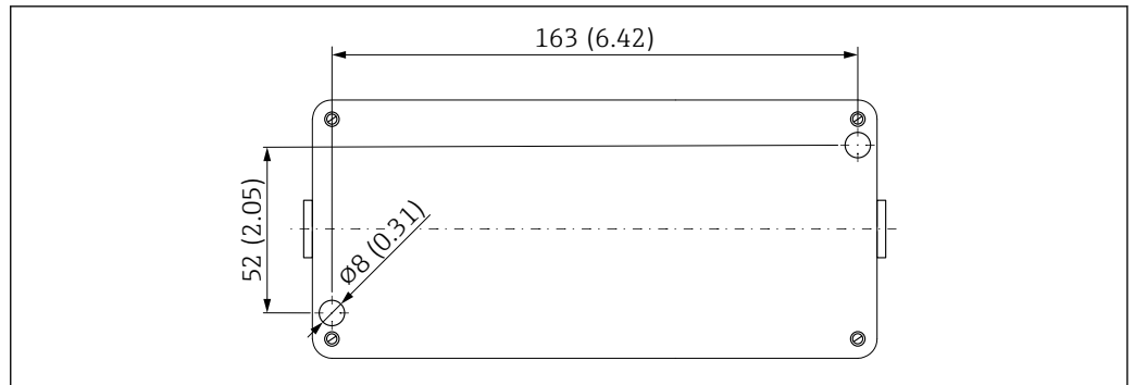
3 Gabarit de montage pour boîtier avec module électronique déporté
