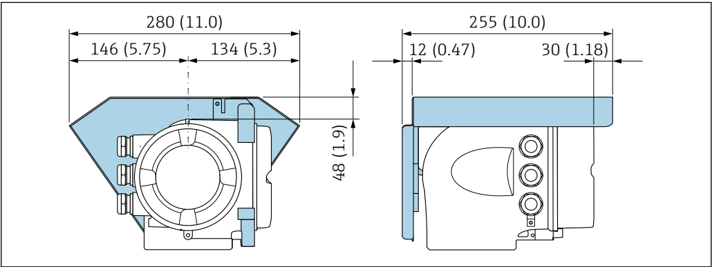
Tapa de protección ambiental
