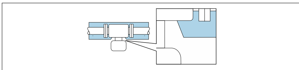
30 Aislamiento térmico con cuello prolongado no aislado
