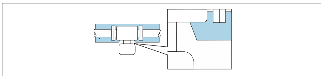
29 Isolation thermique avec tube prolongateur non isolé
