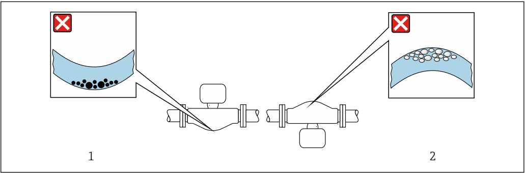
☒ 23 Position du capteur avec tube de mesure coudé
