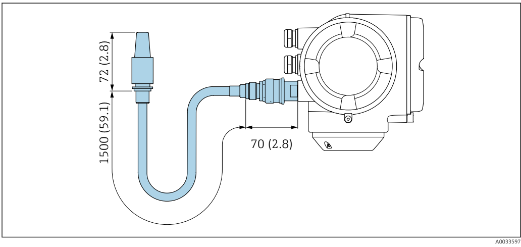
37 Unité de mesure mm (in)
