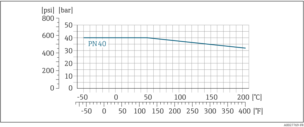
26 Avec matériau de bride 1.4301 (304) ; pièces en contact avec le produit : zirconium 702, tantale
