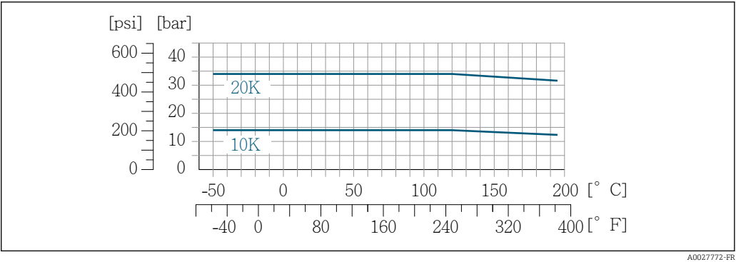
28 Avec matériau de bride 1.4301 (304) ; pièces en contact avec le produit : zirconium 702, tantale
