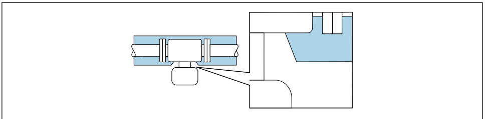
4 Isolation thermique avec tube prolongateur non isolé
