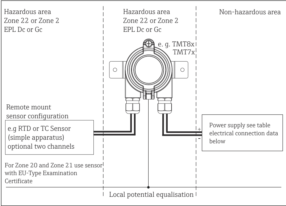
1 Instalación del transmisor para cabezal
