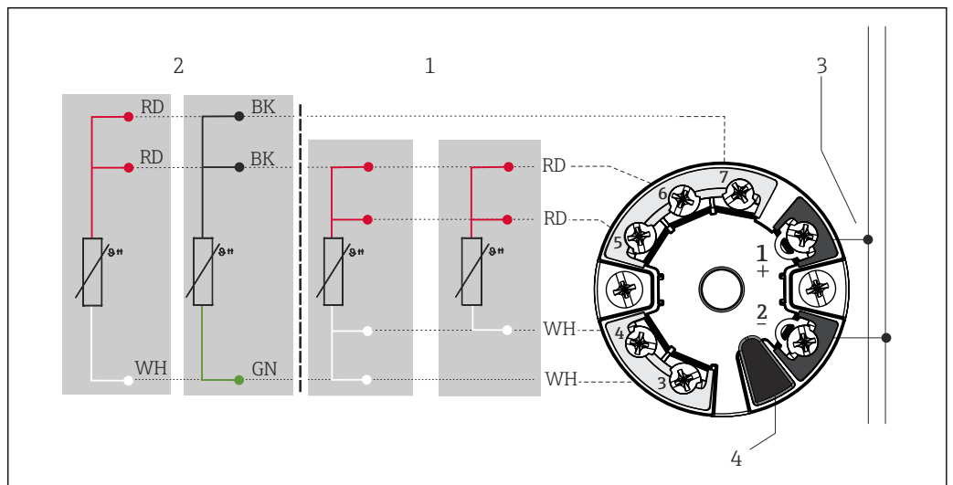
图 4 TMT8x 模块化温度变送器（双输入通道）。如果没有明确要求使用螺纹式接线端子，安装压簧式接线端子。
