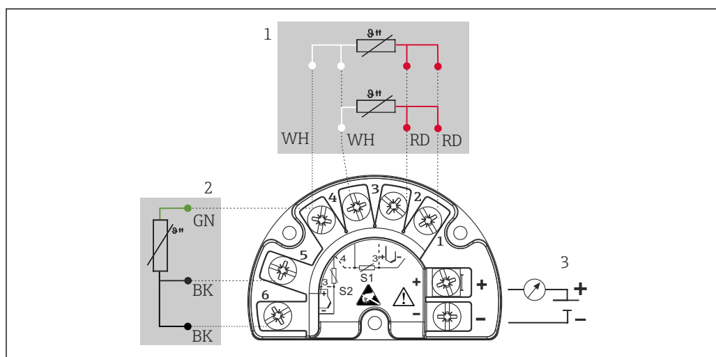
图 6 现场安装的变送器 TMT162（双输入通道）
