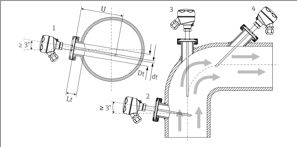
9 安装实例
