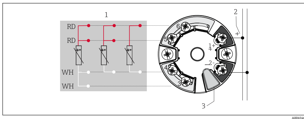
图 5 TMT7x 模块化温度变送器（单输入通道）。如果没有明确要求使用螺纹式接线端子，安装压簧式接线端子。
