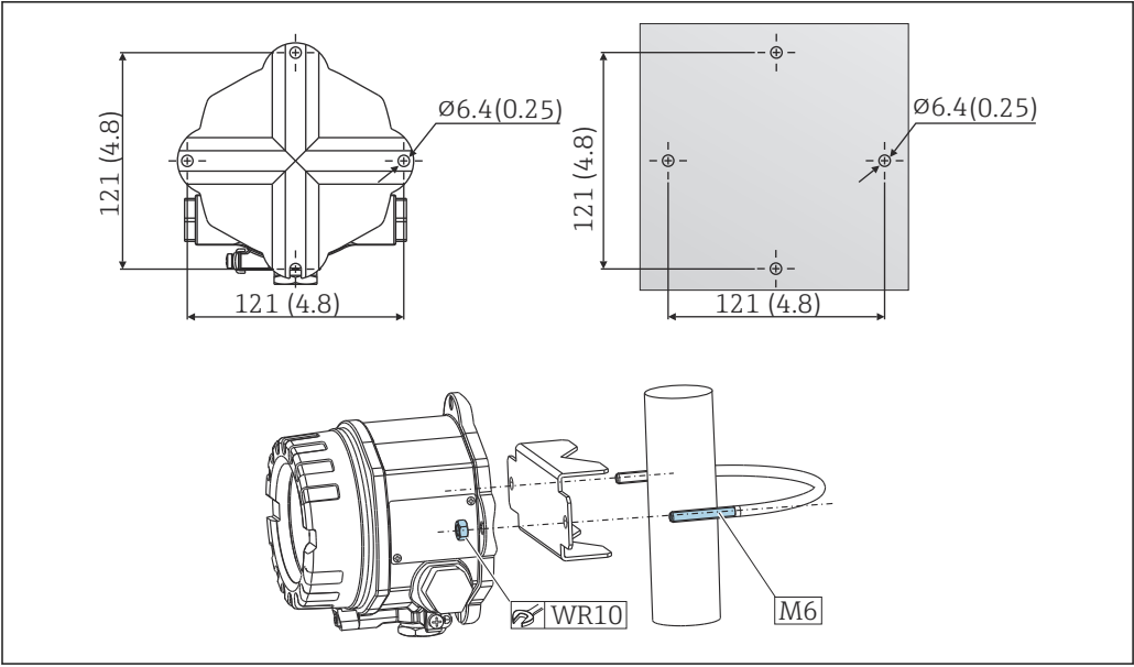
图 2 直接在墙壁上安装现场型变送器，或使用 2"管装架（316L）安装，参见“附件”章节；单位：mm (in)
