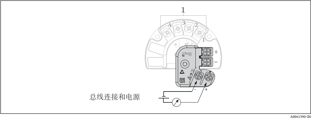
图 9 浪涌保护器的电气连接示意图
