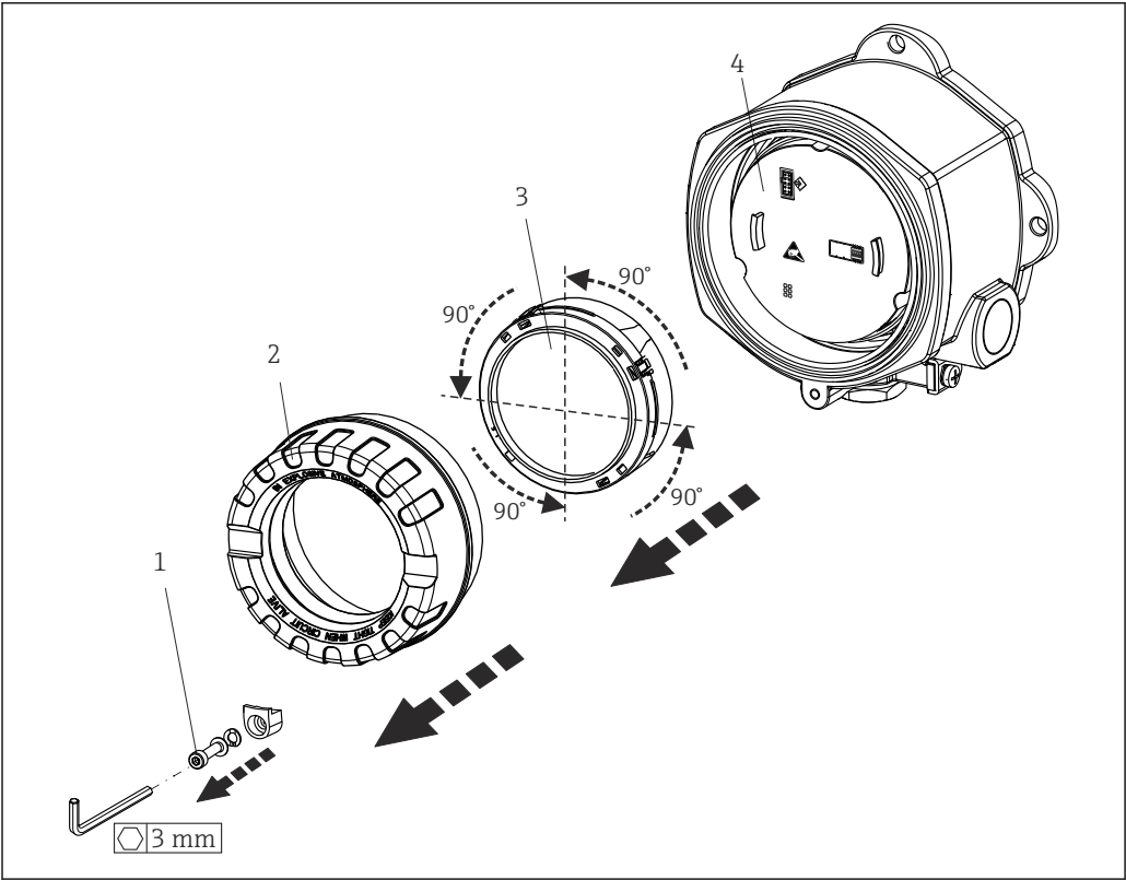
图 3 4 个显示单元固定安装位置，相互间隔 90°
