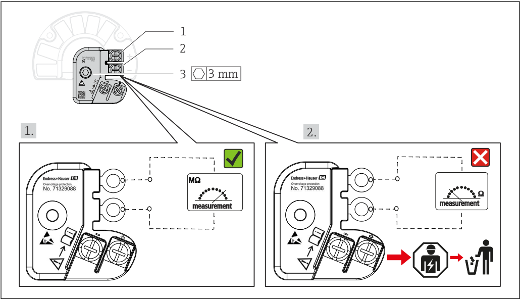
图 10 浪涌保护器的功能测试
