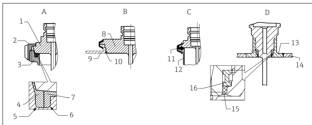
图 3 保证卫生合规的安装指南
