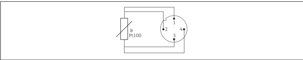
图 6 设备插槽的针脚分配: Pt100, 四线制连接
