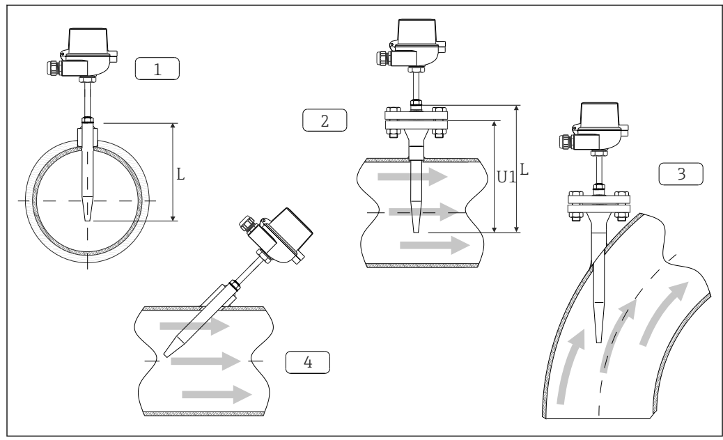
图 8 安装实例
