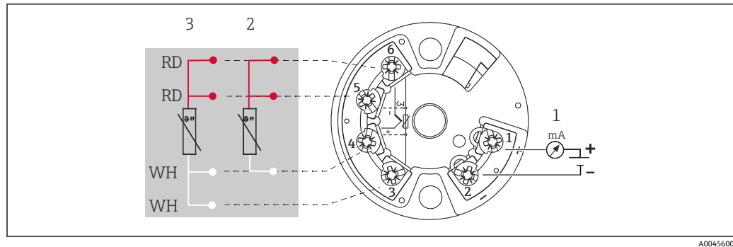
图 4 TMT18x 模块化变送器（单路传感器输入）
