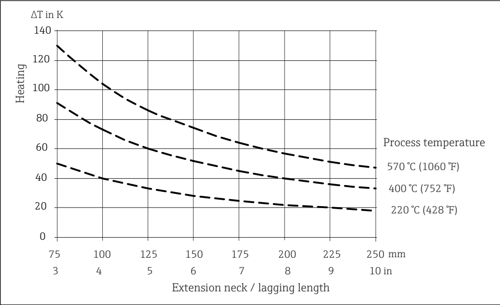
图 9 接线盒温度与过程温度的关系曲线。接线盒温度=环境温度 20 °C (68 °F) + ΔT
