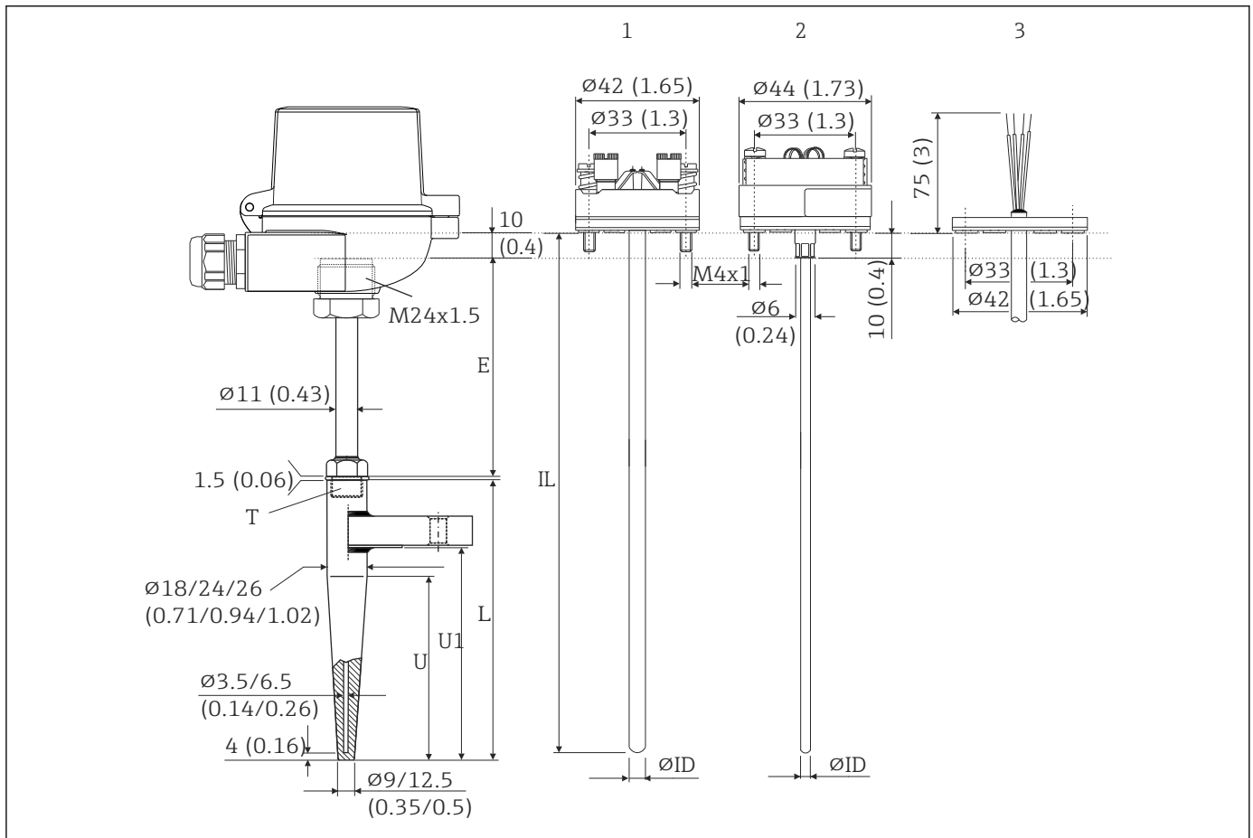
10 TR15 和 TC15 的尺寸
