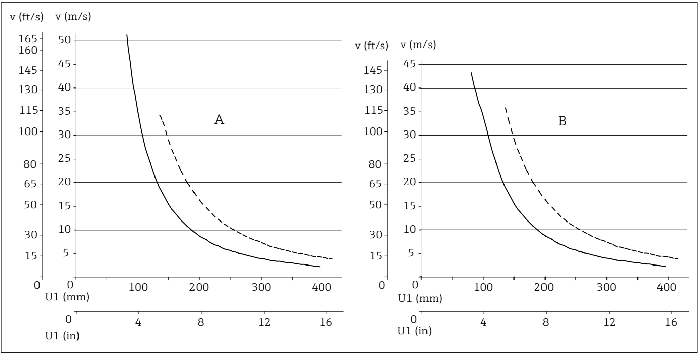
图 7 允许流速，取决于浸入深度
