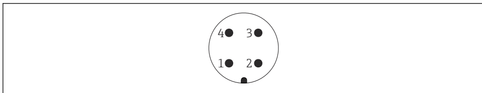
5 Rozmieszczenie styków w gnieździe przyłączeniowym M12
