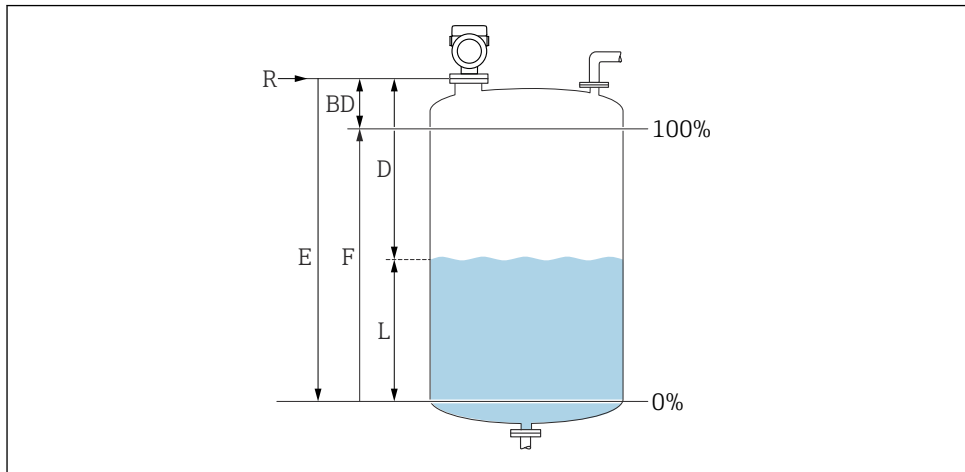
16 Configuratieparameters voor niveaumeting in vloeistof
