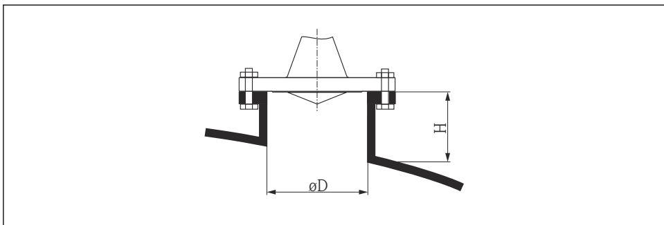
2 Diamètre et hauteur de piquage pour les antennes cornet avec bride tournante
