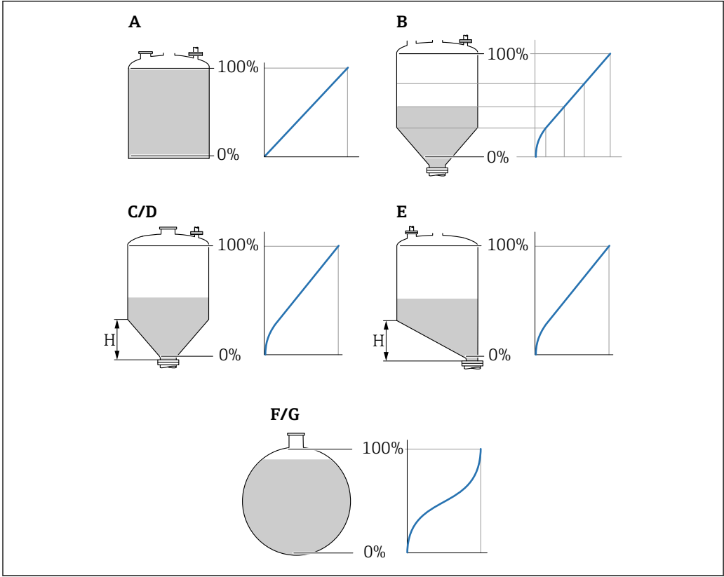
46 Tipos de linealización
