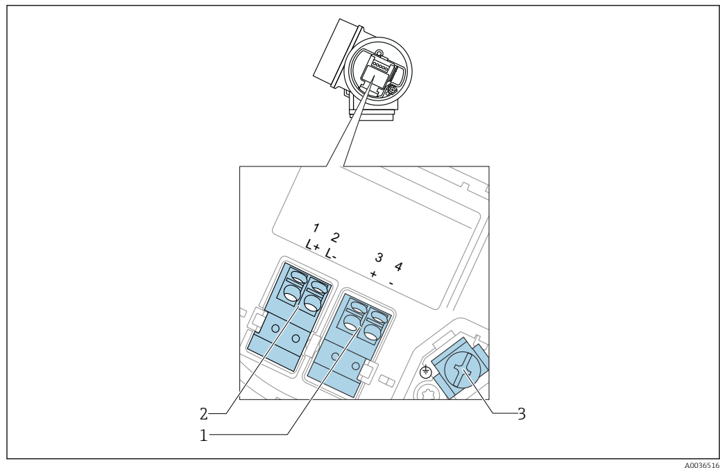
14 Asignación de terminales a cuatro hilos: 4-20 mA HART (10,4 ... 48 V DC )
