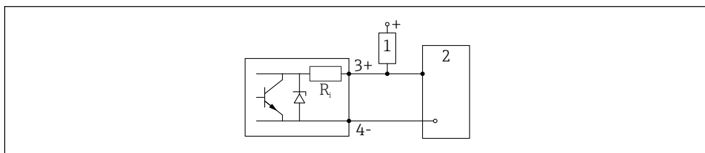
19 Conexión a una entrada digital
