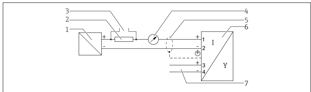
11 Diagrama en bloque a dos hilos: 4-20 mA HART, salida de conmutación
