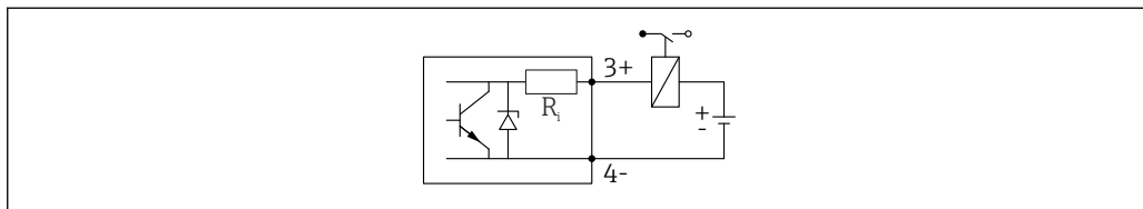
18 Conexión de un relé
