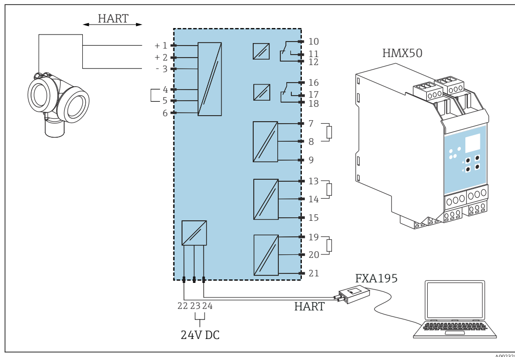
20 Diagrama de conexión del convertidor de lazo HART HMX50 (ejemplo: instrumento pasivo a 2 hilos y salidas de corriente conectados como fuentes de alimentación)
