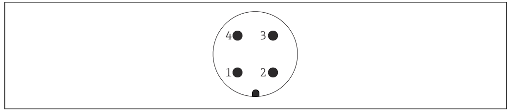
21 Asignación de pines del conector M12
