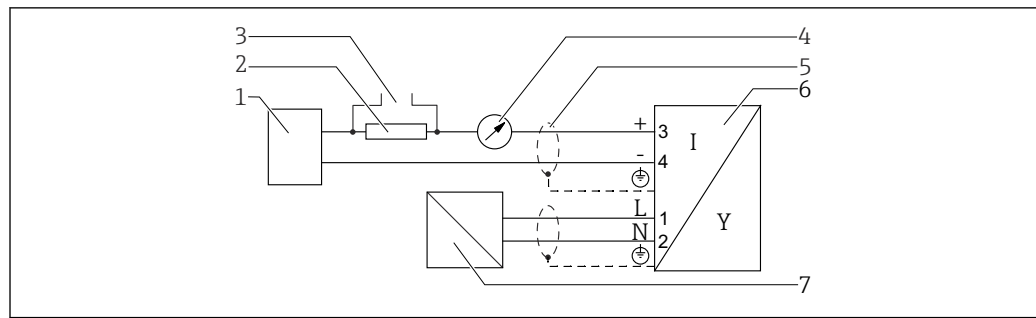
17 Diagrama en bloque a cuatro hilos: 4-20 mA HART (90 ... 253 V AC )
