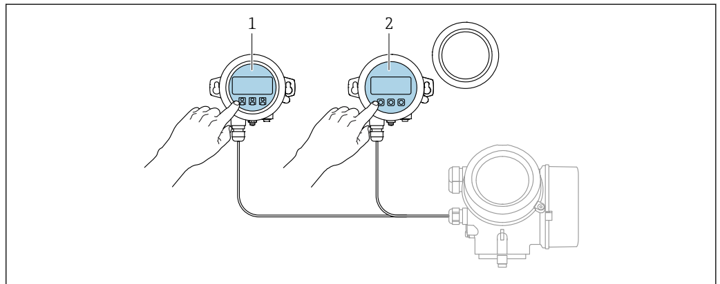
25 Modos de configuración con FHX50
