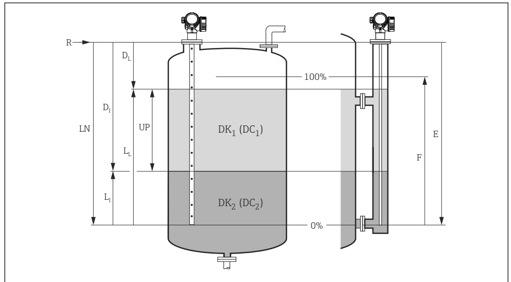
35 Parámetros de configuración para la medición de la interfase
