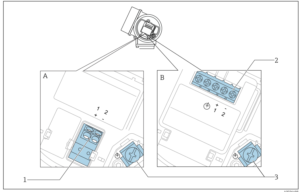
8 Asignación de terminales a 2 hilos: 4-20 mA HART
