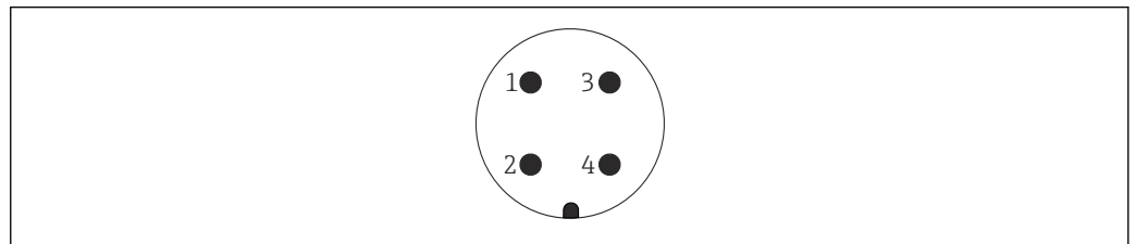
22 Asignación de pines del conector 7/8"
