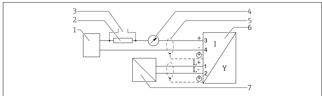
15 Diagrama en bloque a cuatro hilos: 4-20 mA HART (10,4 ... 48 V DC )
