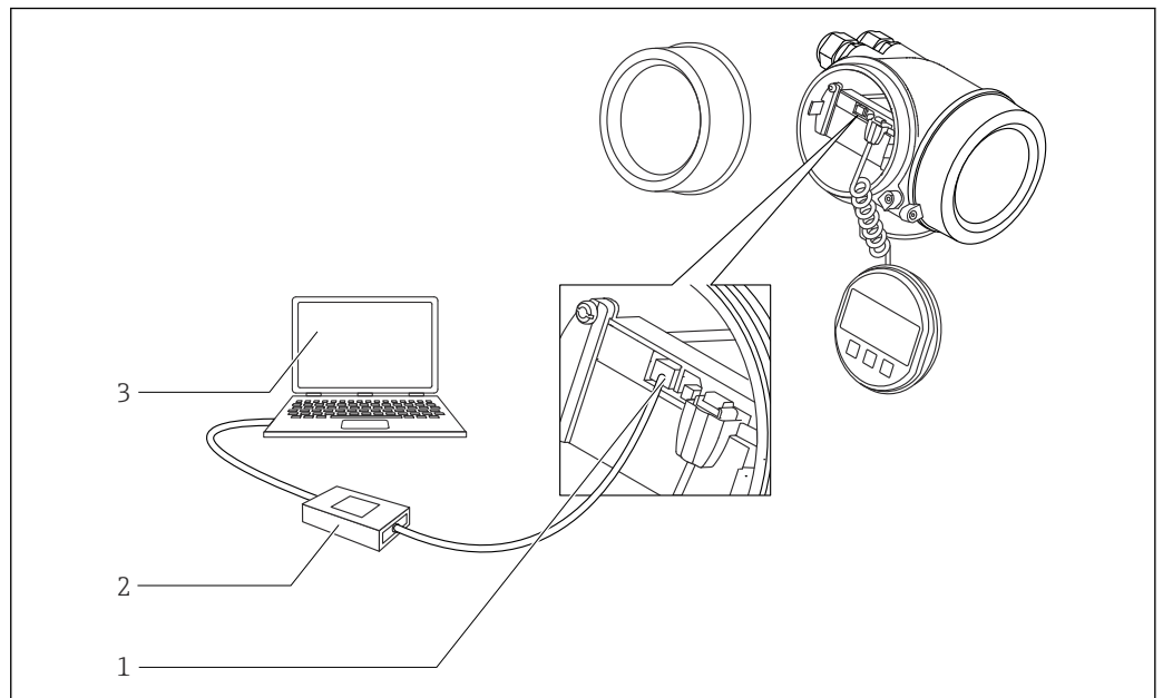
29 DeviceCare/FieldCare mediante interfaz de servicio (CDI)
