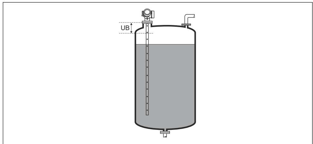
47 Distancia de bloqueo (UB) para mediciones de líquidos
