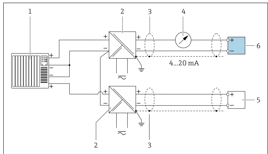
図 10 マイナスコモン HART 入力 (パッシブ) の接続例
