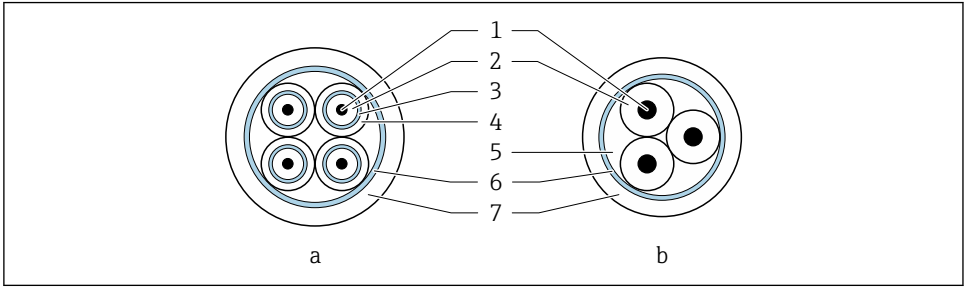
☐ 3 케이블 단면
