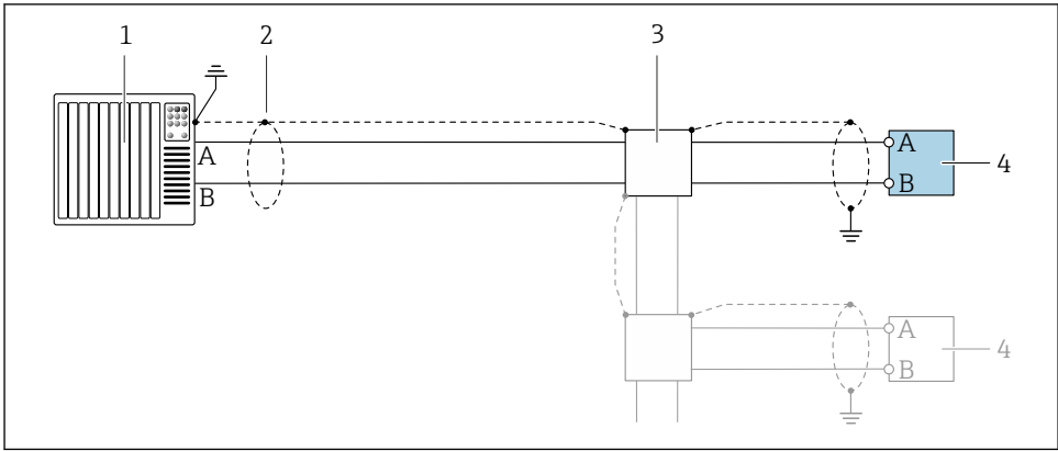
☐ 5 Modbus RS485의 연결 예시, 비방폭 지역 및 Zone 2/Class I/Division 2
