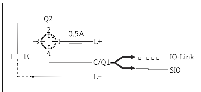
Pin 1 Voedingsspanning +
