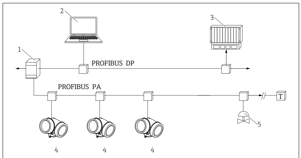
16 Options de configuration à distance via protocole PROFIBUS PA
