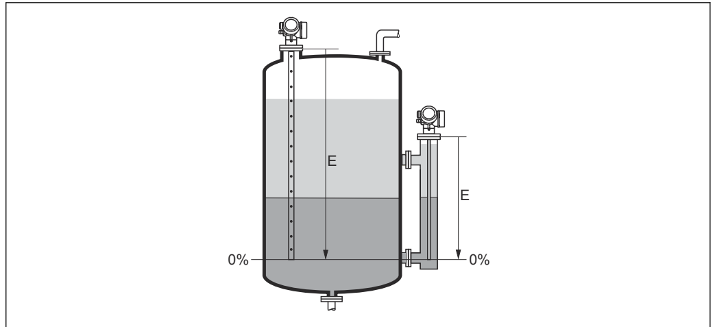
29 Distance du point zéro (E) pour la mesure d'interface
