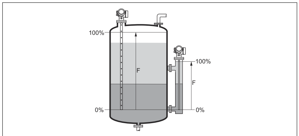
30 Plage de mesure (F) pour la mesure d'interface
