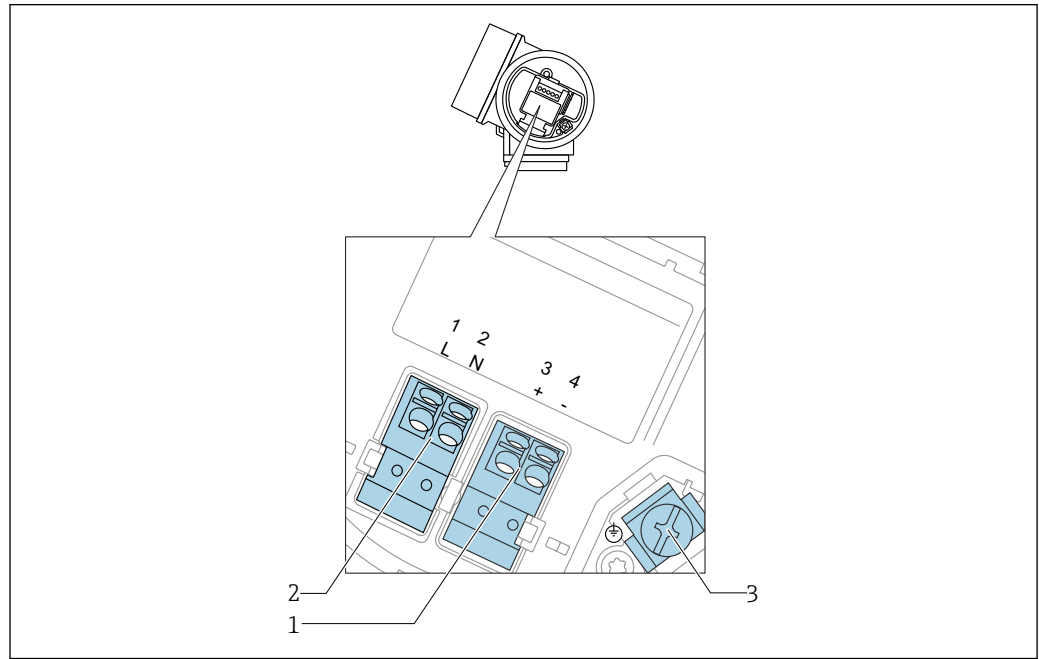
8 Occupation des bornes 4 fils : 4-20mA HART (90 ... 253 V AC )
