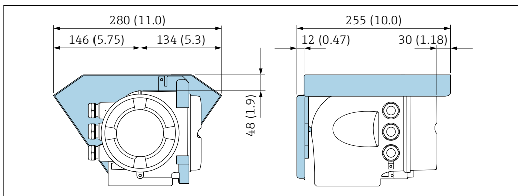
9 Unité de mesure mm (in)
