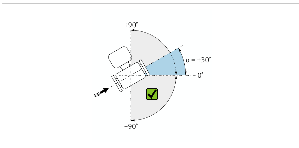
7 Vue latérale avec le sens d'écoulement de gauche à droite.
