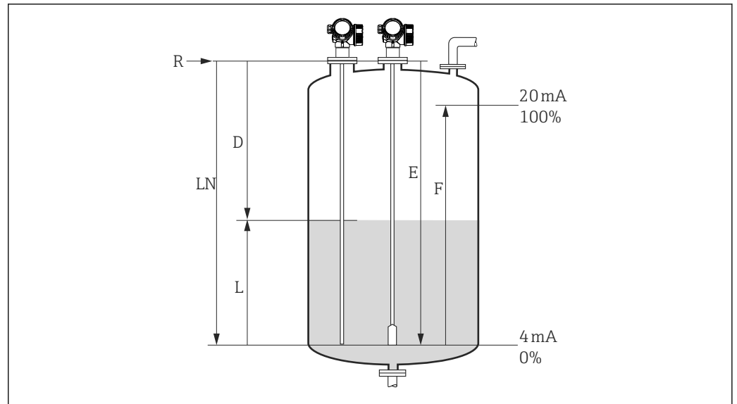
图 23 液位测量时的设置参数
