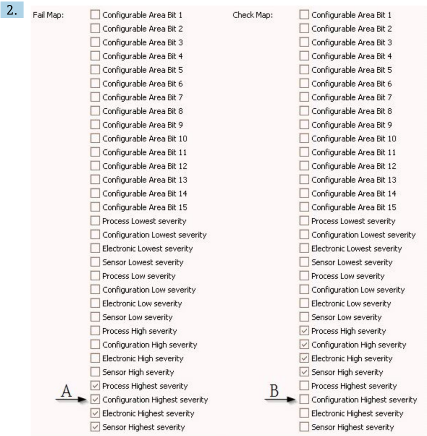
图 27 “故障抑制”和“检查抑制”栏的缺省设置。
