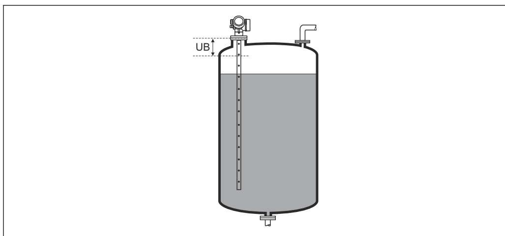
41 液位测量的盲区距离 (UB)
