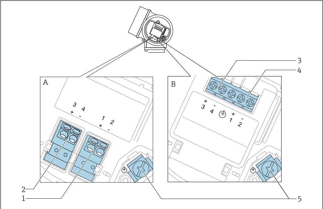
图 10 接线端子分配: PROFIBUS PA / FOUNDATION Fieldbus
