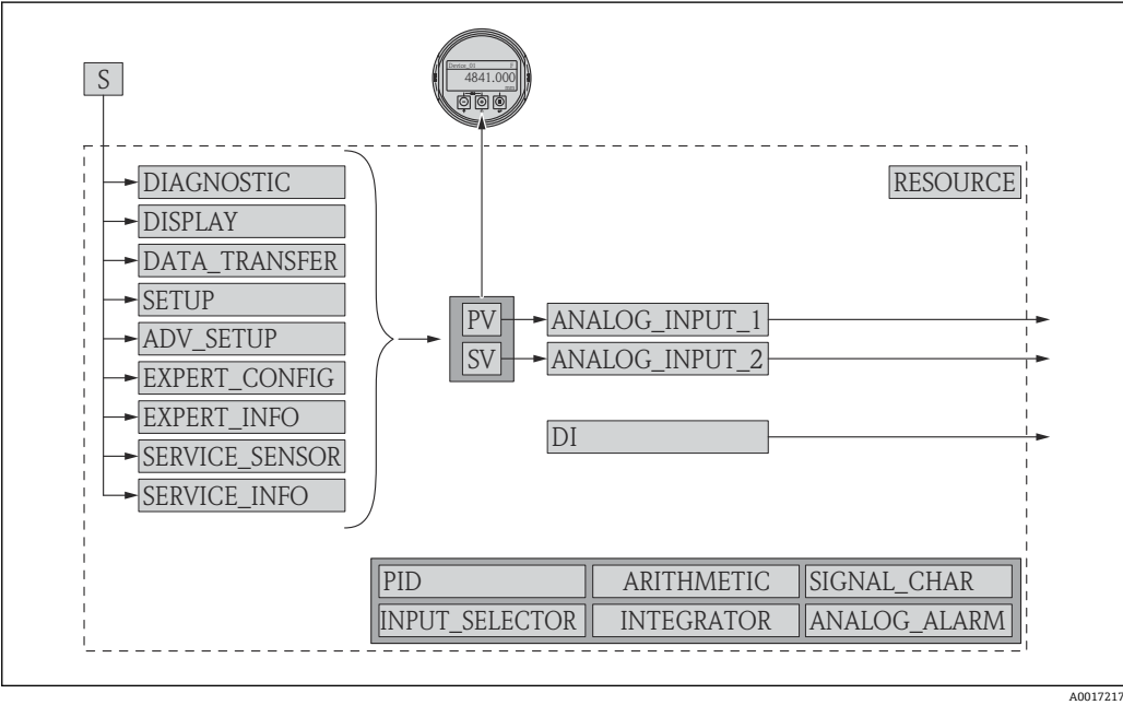
图 21 设备块的出厂设置 S 传感器 PV 主要测量值：物位（或线性化值） SV 第二测量值：距离
