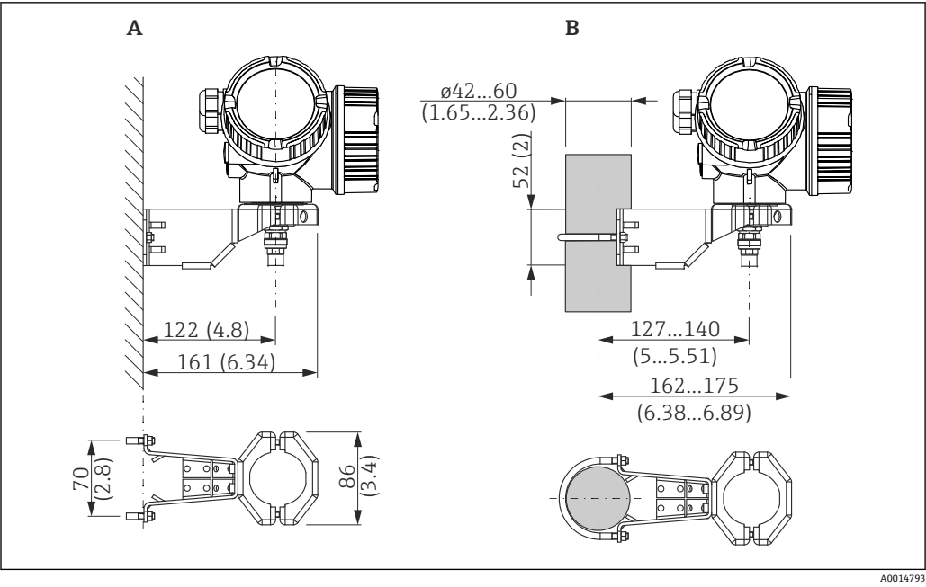
图 7 使用安装支架安装电子腔外壳；单位：mm (in) A 墙装 B 管装
