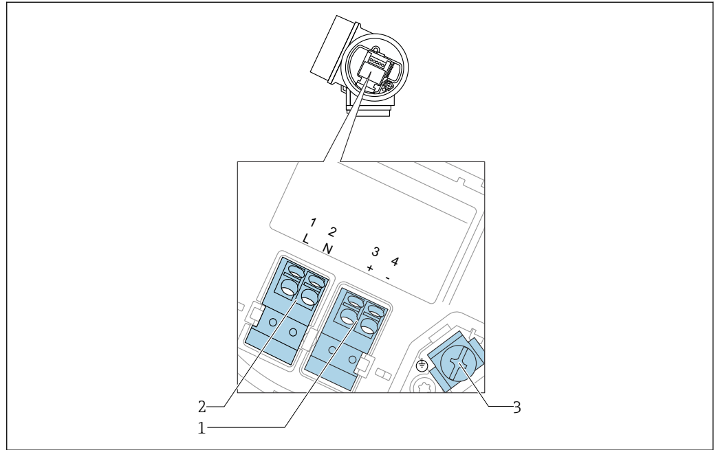
图 9 接线端子分配：四线制；4...20 mA HART (90 ... 253 V AC )
