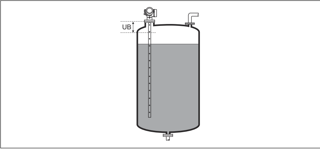
图 38 液位测量的盲区距离 (UB)
