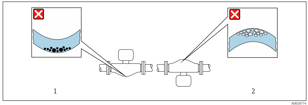
23 Orientación del sensor con tubo de medición curvado
