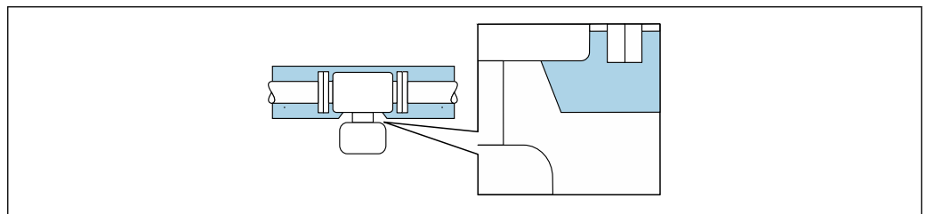
28 Aislamiento térmico con cuello prolongado no aislado
