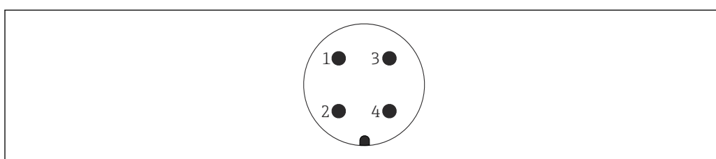
20 Asignación de pins del conector 7/8"
