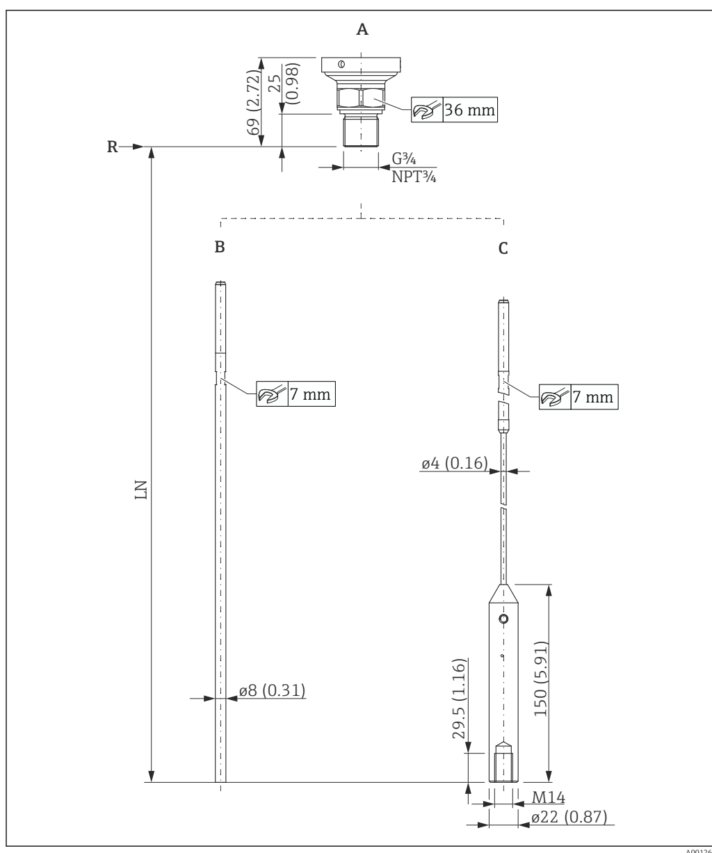
31 FMP50: Conexión a proceso / sonda. Unidad de medida mm (in)
