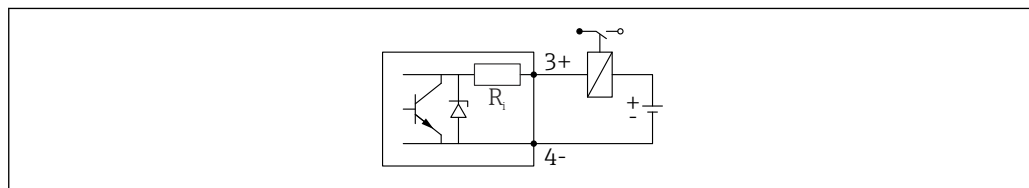
17 Conexión de un relé
