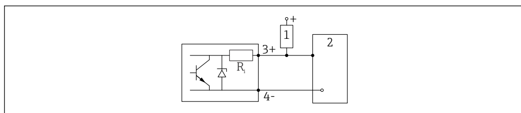
18 Conexión a una entrada digital
