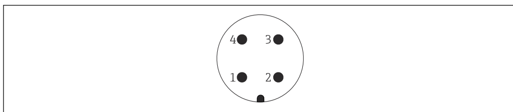
19 Asignación de pins del conector M12
