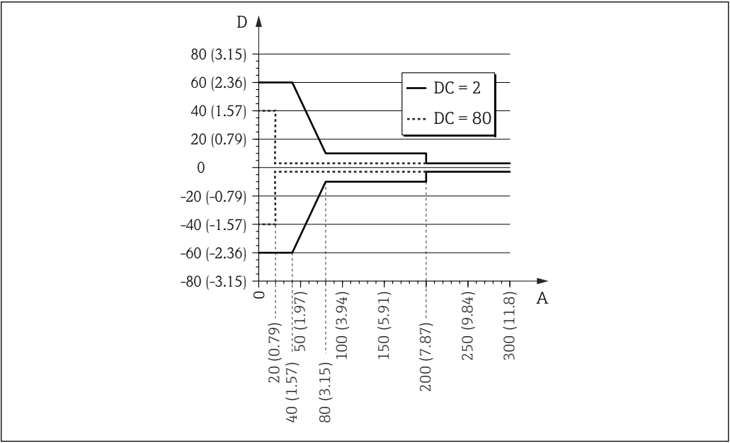
21 Error medido en el extremo de la sonda para sondas de varilla y coaxiales
