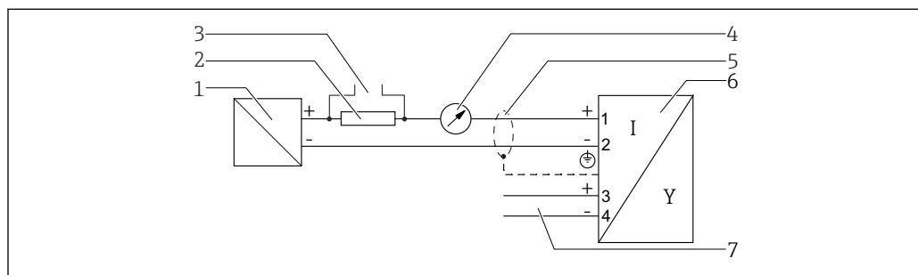
图 15 接线图：两线制；4...20 mA HART，开关量输出
