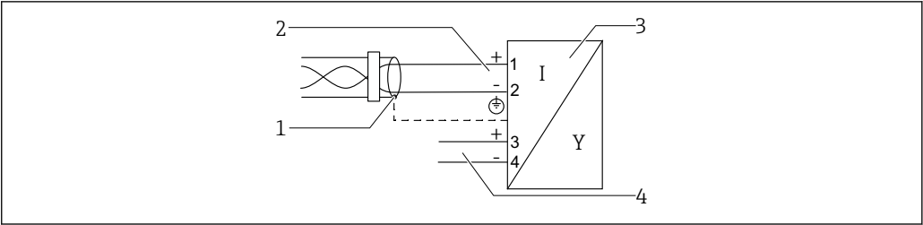
23 接线图: PROFIBUS PA / FOUNDATION Fieldbus
