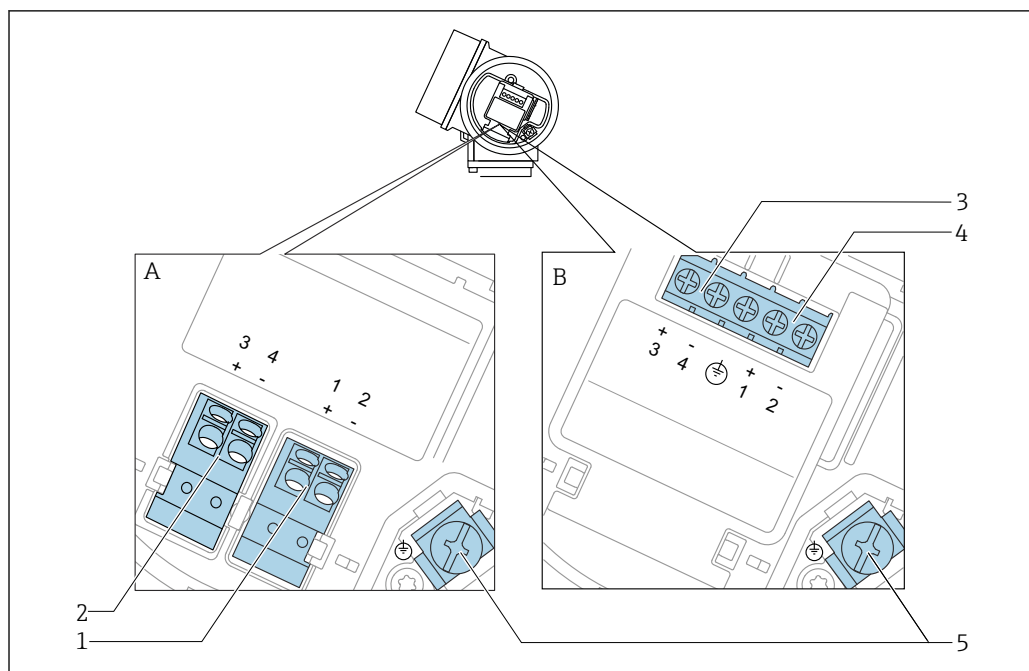
图 14 接线端子分配：两线制；4...20 mA HART，开关量输出
