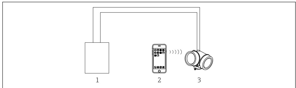
图 53 通过 SmartBlue (app) 操作
