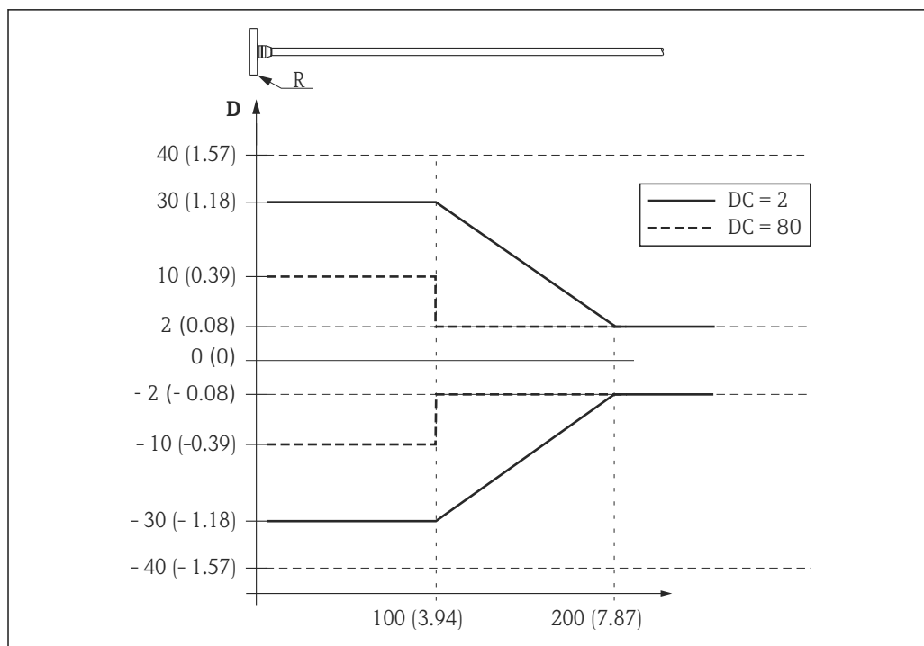
图 32 探头顶部出现的测量误差；单位：mm (in)
