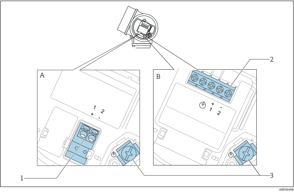
12 接线端子分配：两线制；4...20 mA HART
