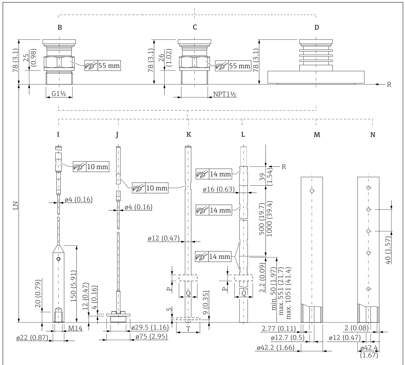
47 FMP51: 过程连接和探头。测量单位 mm (in)
