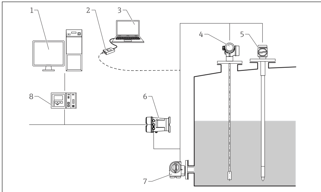
图 58 完整的测量系统包括：
