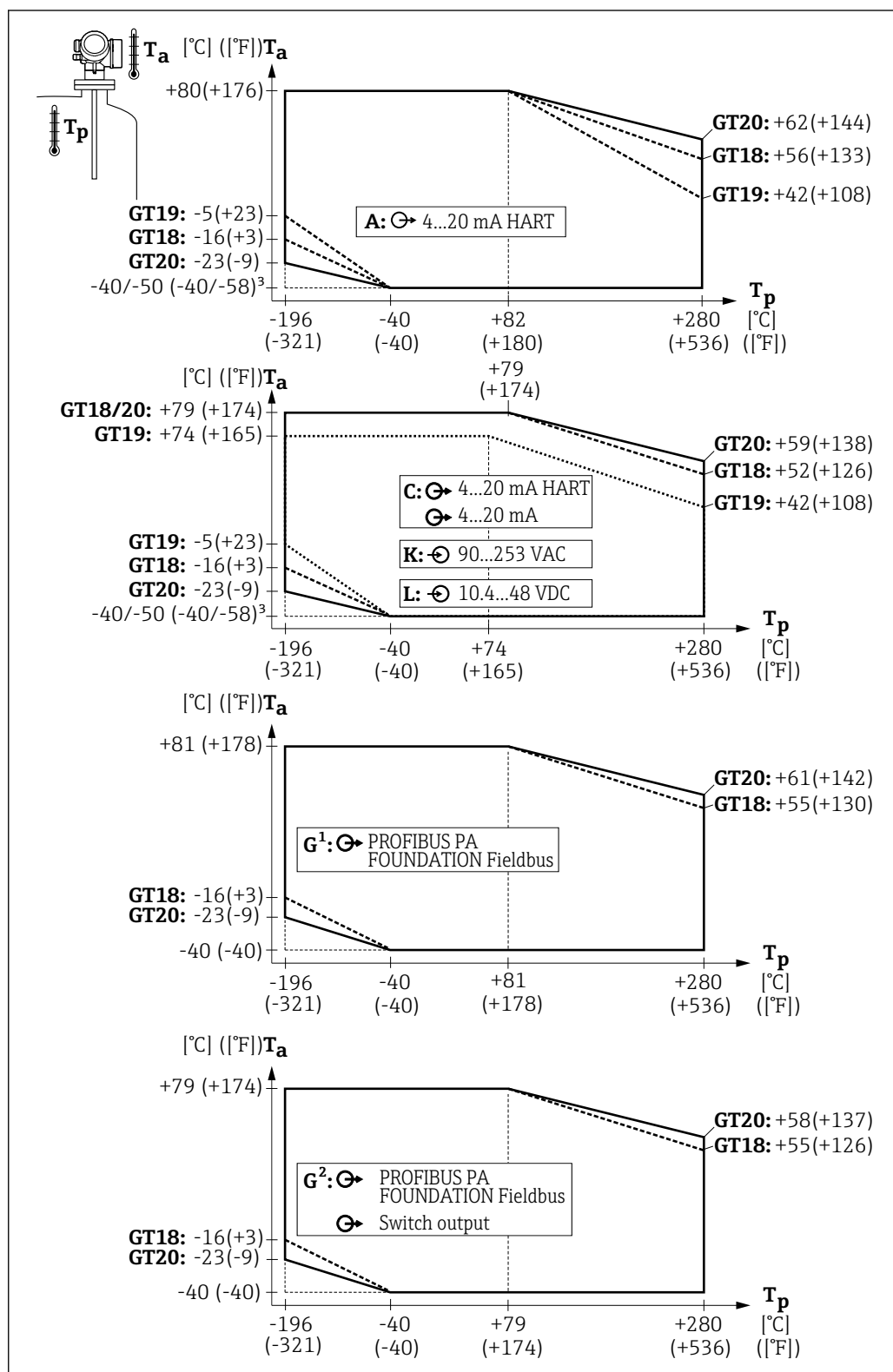
温度曲线: FMP54, 增温型 (XT), 最高+280 °C (+536 °F)
