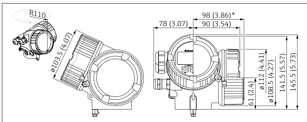
图 43 GT20 外壳 (铝, 带涂层)。测量单位 mm (in)
