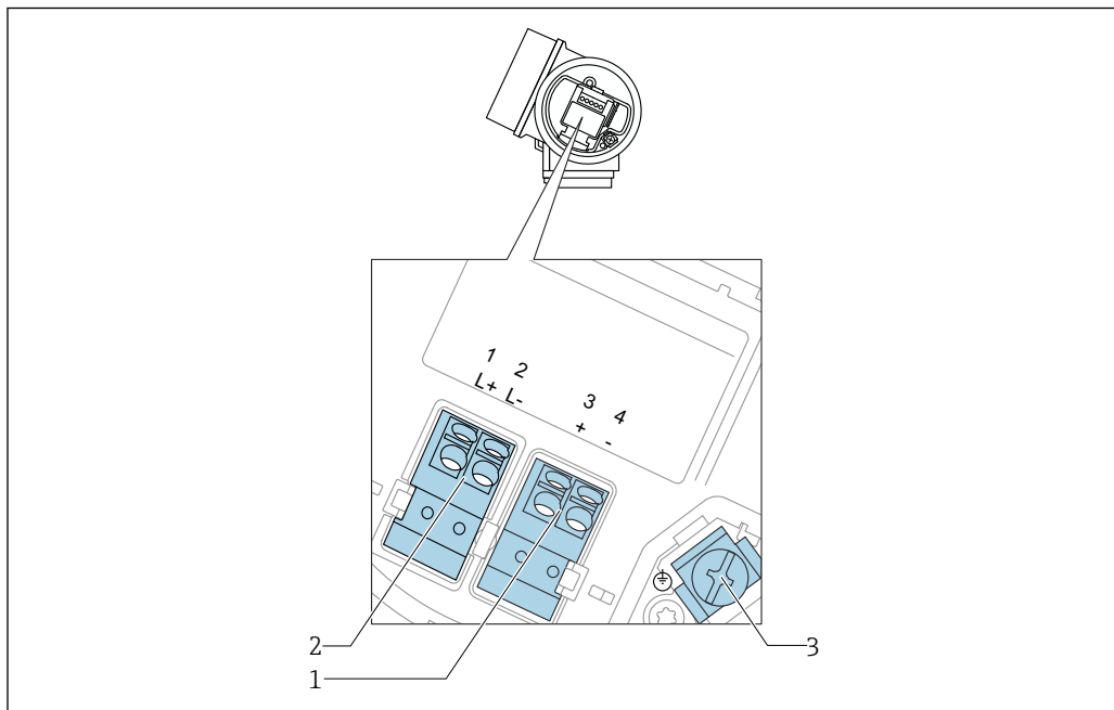
图 18 接线端子分配：四线制；4...20 mA HART (10.4 ... 48 V DC )
