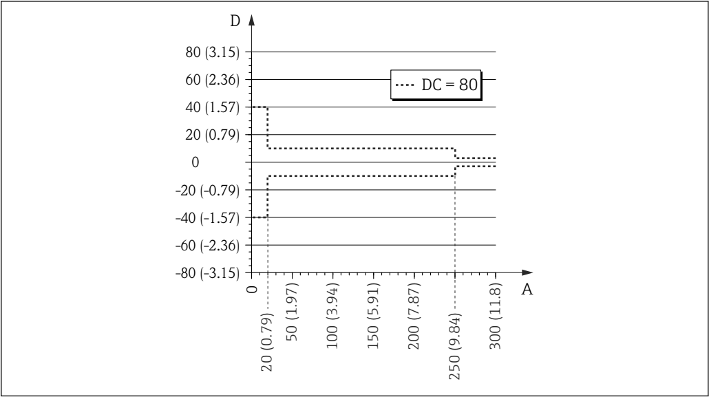
30 缆式探头底部的测量误差
