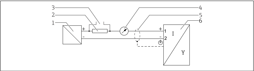
13 接线图：两线制；4...20 mA HART
