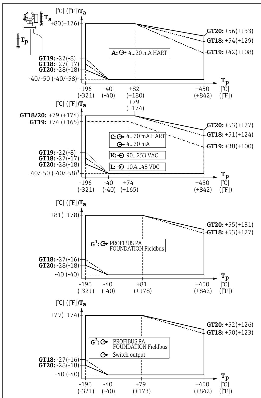
温度曲线: FMP54, 高温型 (HT) , 最高+450 °C (+842 °F)
