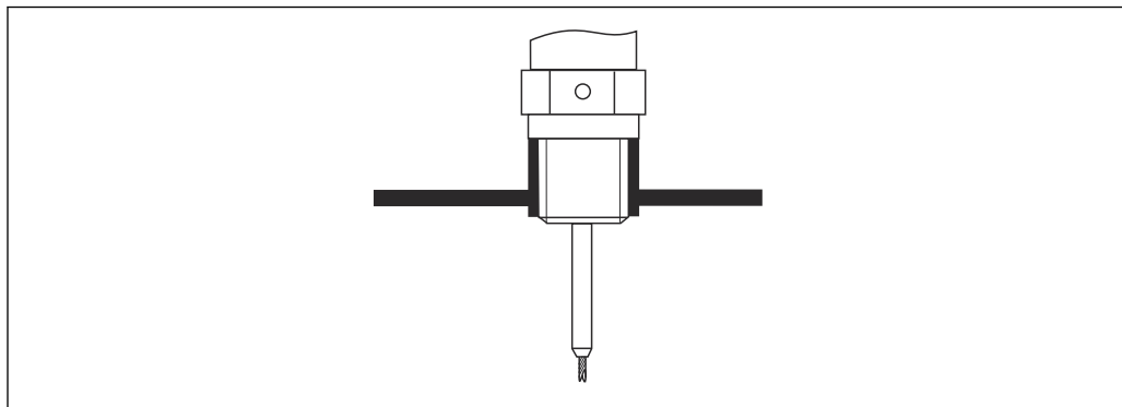
图 35 安装带螺纹连接的仪表；与罐顶齐平安装
