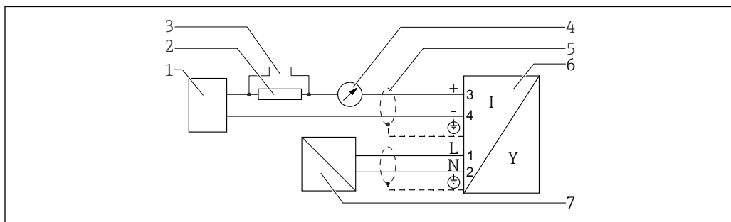
图 21 接线端子分配：四线制；4...20 mA HART (90 ... 253 V AC )
