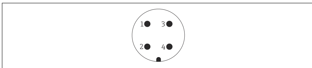
图 28 7/8"插头的针脚分配
