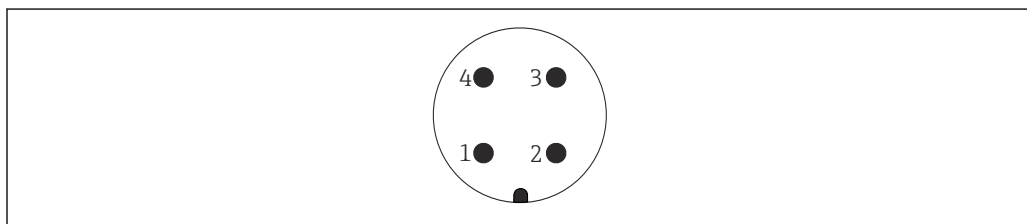
图 27 M12 插头的针脚分配
