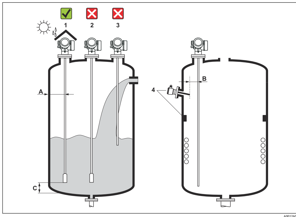
图 34 Levelflex 的安装条件
