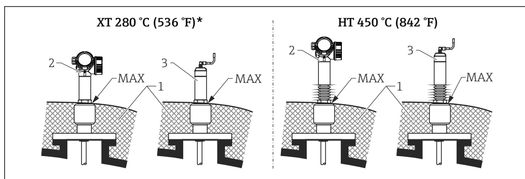
图 40 法兰过程连接 - 增温型 (XT) 和高温型 (HT) 仪表
