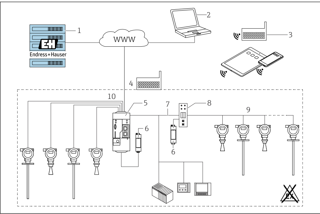
图 60 SupplyCare Hosting SCH30 的库存管理平台示例
