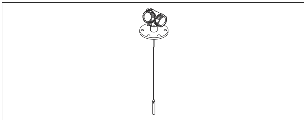
图 7 带定心杆的缆式探头
