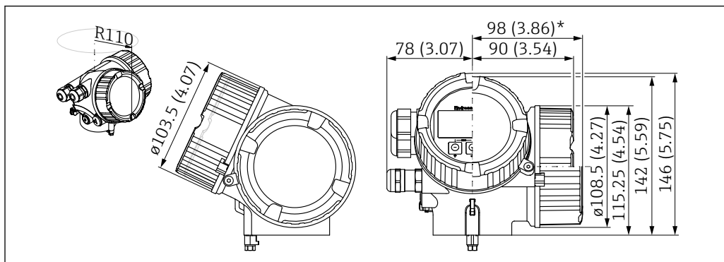
图 41 GT18 外壳 (316 L)。测量单位 mm (in)
