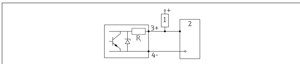
图 25 连接数字量输入
