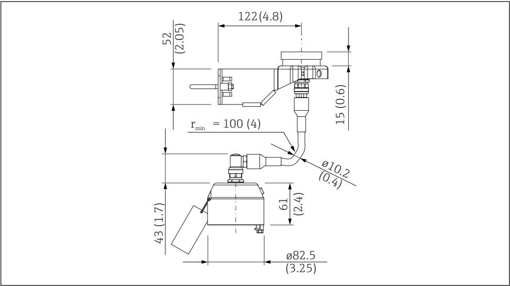
图 45 分体式探头的连接尺寸；连接电缆长度为订购长度。测量单位 mm (in)
