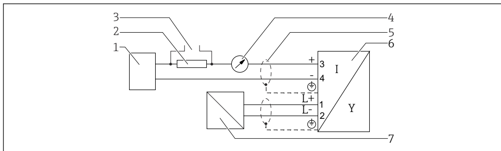
图 19 接线端子分配：四线制；4...20 mA HART (10.4 ... 48 V DC )
