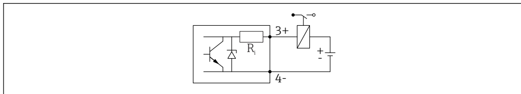
图 24 连接继电器
