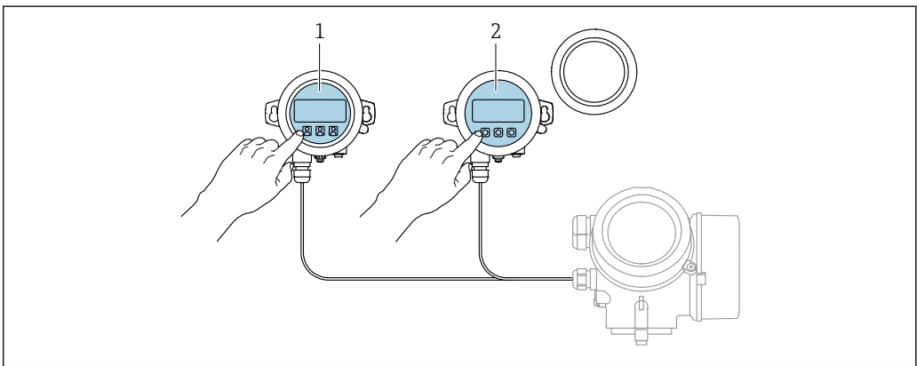
图 51 FHX50 的操作选项
