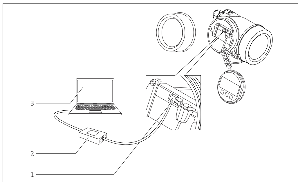
图 49 DeviceCare/FieldCare, 使用服务接口 (CDI)
