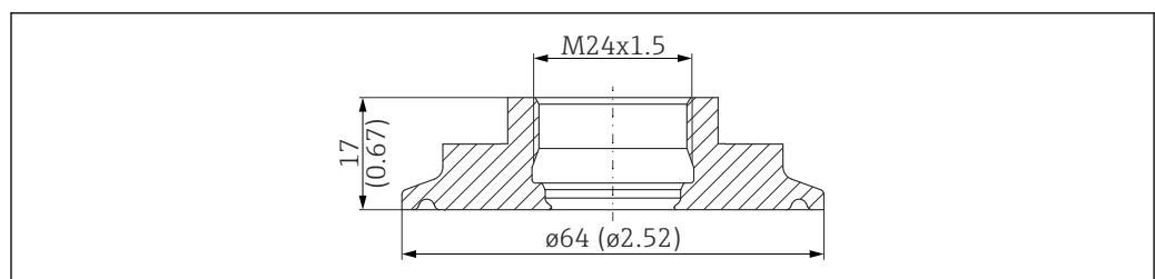
35 Tri-Clamp ISO2852 DN40...51 (2") 卡箍, 316L。测量单位 mm (in)
