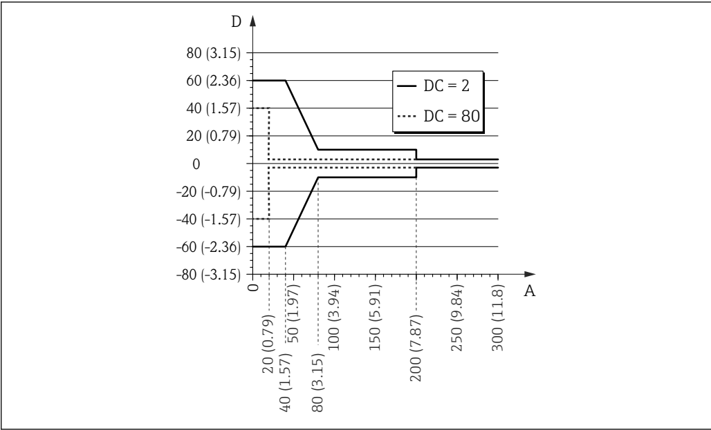
20 杆式探头和同轴探头底部附近的测量误差
