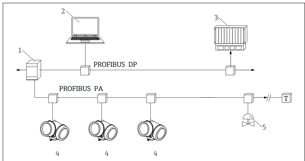
图 47 通过 PROFIBUS PA 网络进行远程操作
