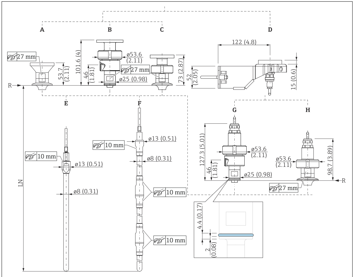
42 FMP53: 探头。测量单位 mm (in)
