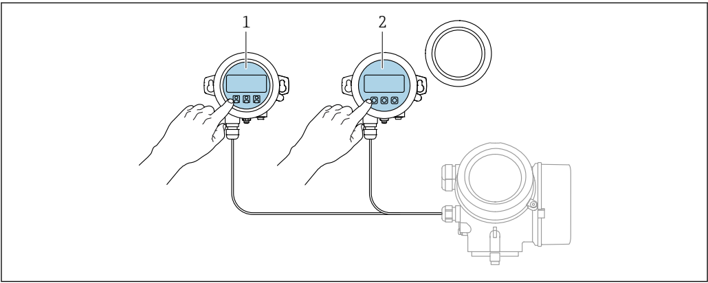
43 FHX50 的操作选项 1 显示与操作单元 SD03, 光敏键操作, 可以在玻璃盖板外部操作 2 显示与操作单元 SD02, 按键操作; 必须打开盖板
