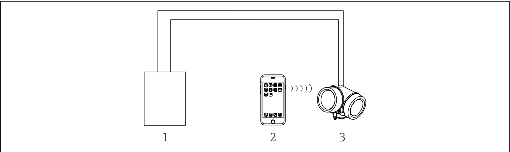
45 通过 SmartBlue (app) 操作
