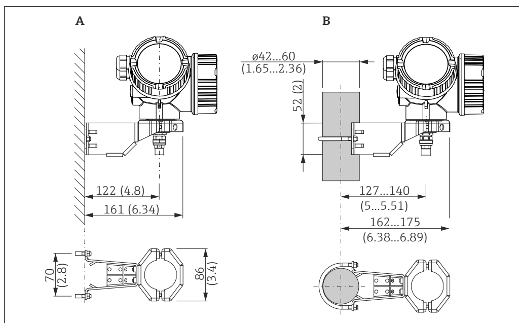
26 电子腔外壳安装架。测量单位 mm (in)
