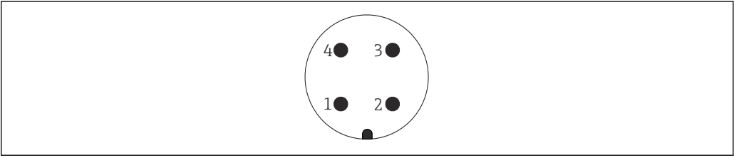
图 18 M12 插头的针脚分配
