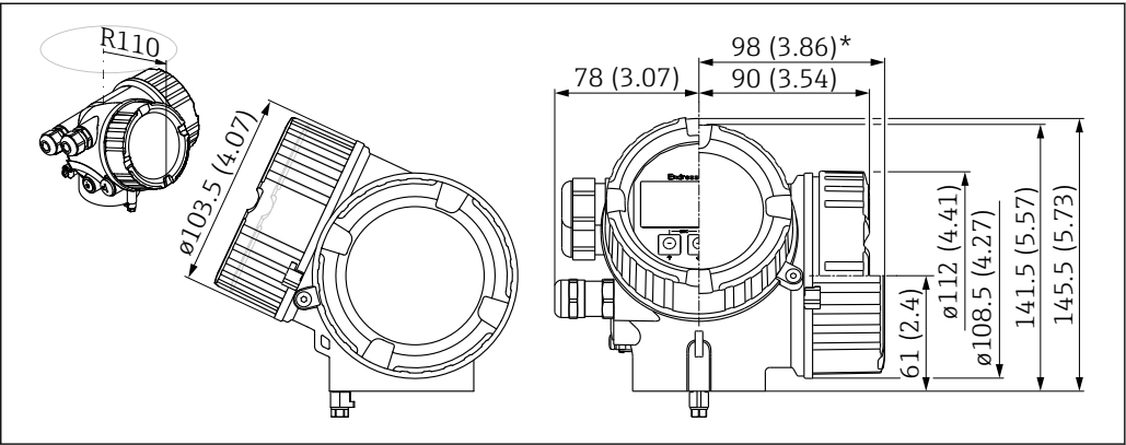
图 25 GT20 外壳（铝，带涂层）。测量单位 mm (in)
