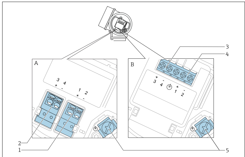
图 14 接线端子分配：PROFIBUS PA / FOUNDATION Fieldbus
