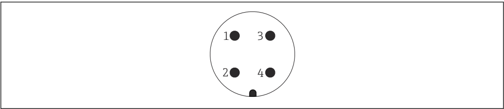
图 19 7/8"插头的针脚分配
