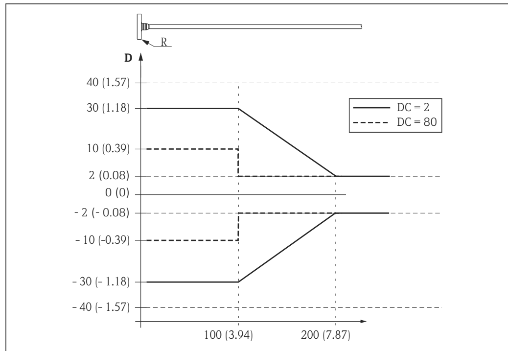
图 21 探头顶部出现的测量误差；单位：mm (in)
