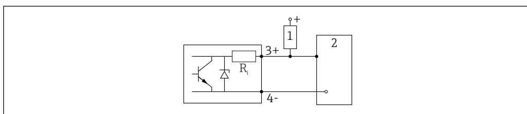
图 17 连接数字量输入
