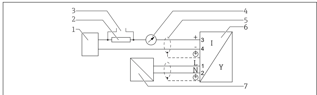
图 13 接线端子分配：四线制；4...20 mA HART (90 ... 253 V AC )
