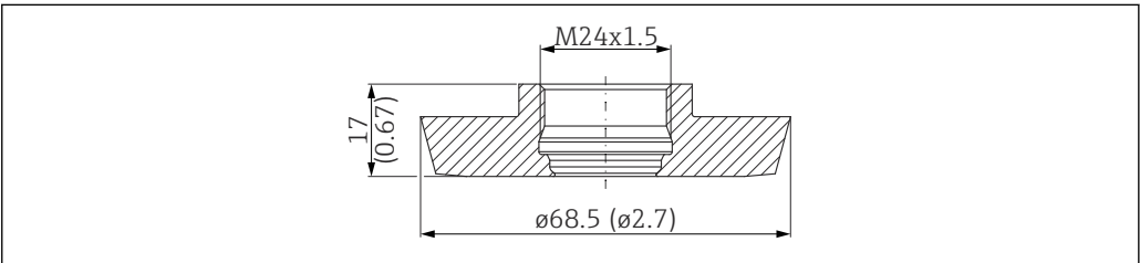
30 DIN11851 DN40 开槽螺母, PN25, 316L。测量单位 mm (in)
