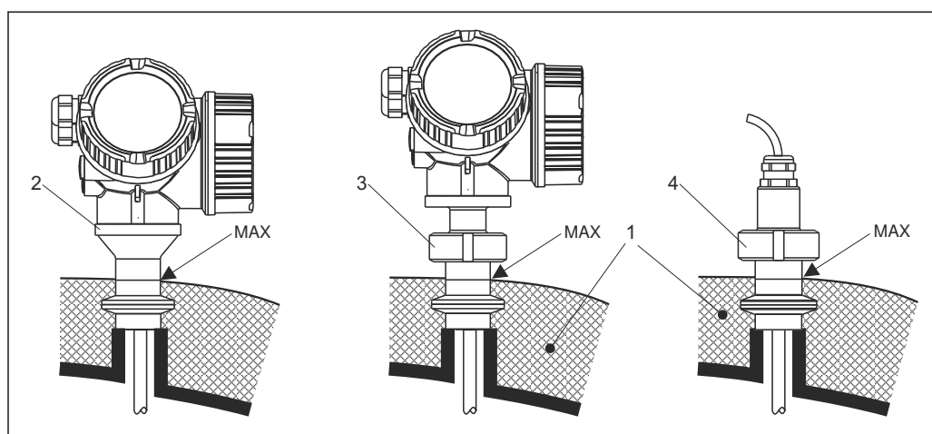
23 卫生型过程连接
