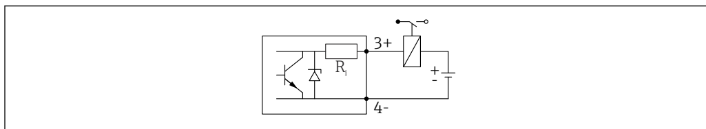
图 16 连接继电器
