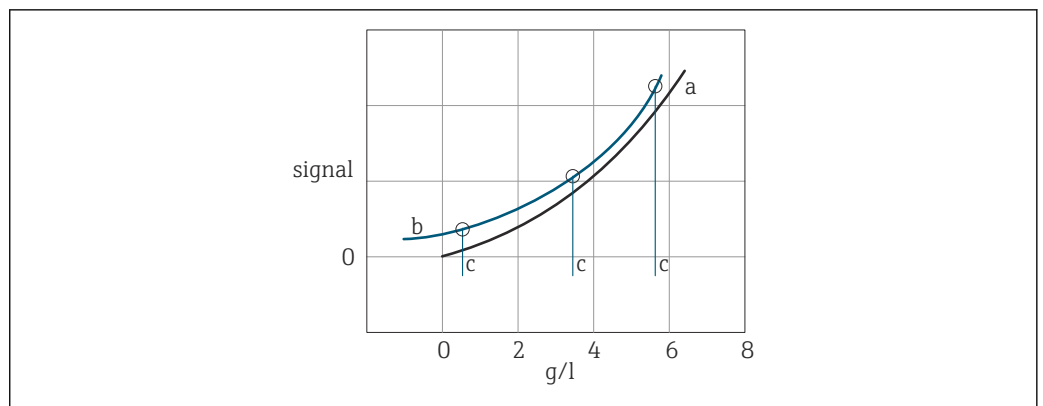
31 Calibrado a tres puntos
