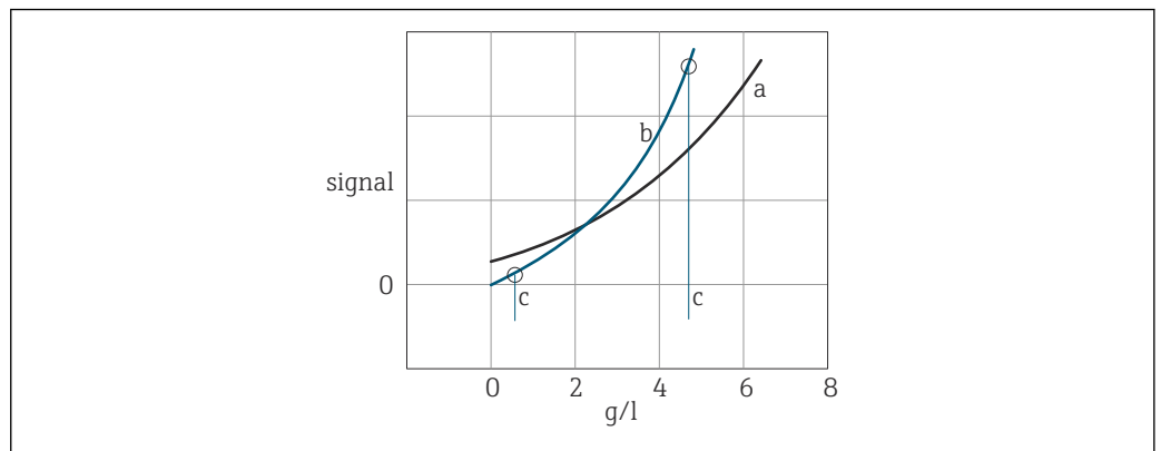
30 Calibración a dos puntos
