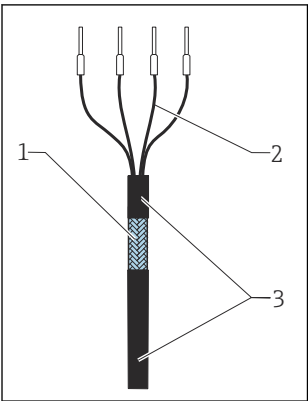
24 Cable terminado 1 Blindaje externo (a la vista) 2 Hilos del cable con terminales de empalme 3 Cubierta del cable (aislante)
