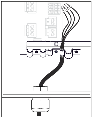
26 Apretar el tornillo (2 Nm (1,5 lbf ft)) El blindaje del cable se pone a tierra mediante la presilla
