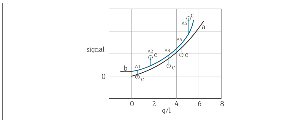
32 Calibración a cinco puntos
