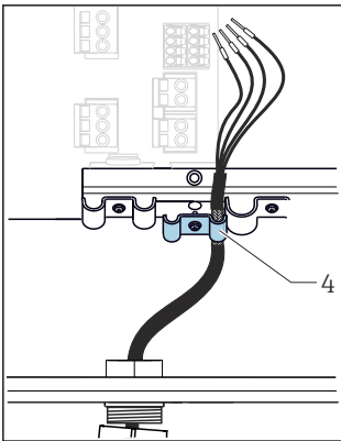
25 Inserción del cable 4 Presilla de puesta a tierra
