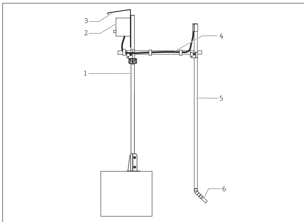
10 Sistema de medición con portasondas de inmersión (ejemplo)
