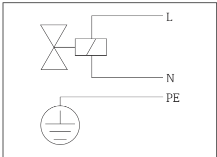
10 Schéma de principe système de préparation d'échantillons, Liquiline System CAT810 avec vanne de nettoyage
