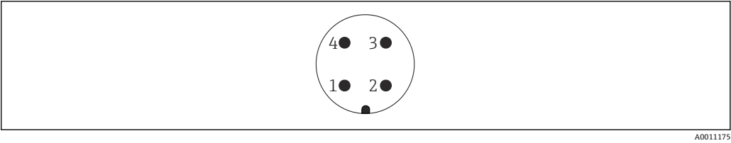
图 3 仪表上的连接插头
