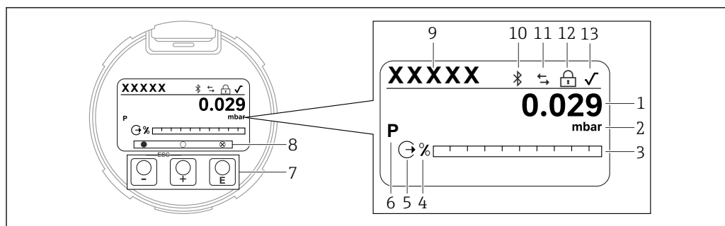
图 9 图形显示屏，带光敏按键。
