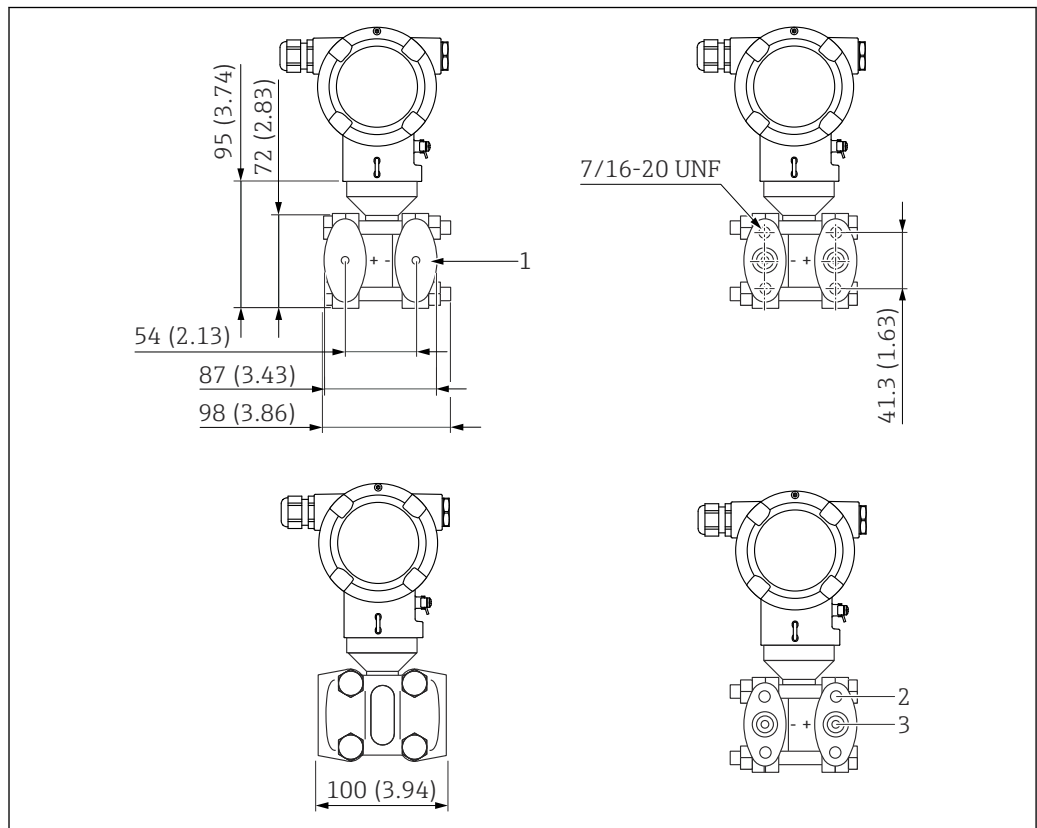
4 正视图、左视图、右视图。螺母始终安装在负压侧。测量单位 mm (in)
