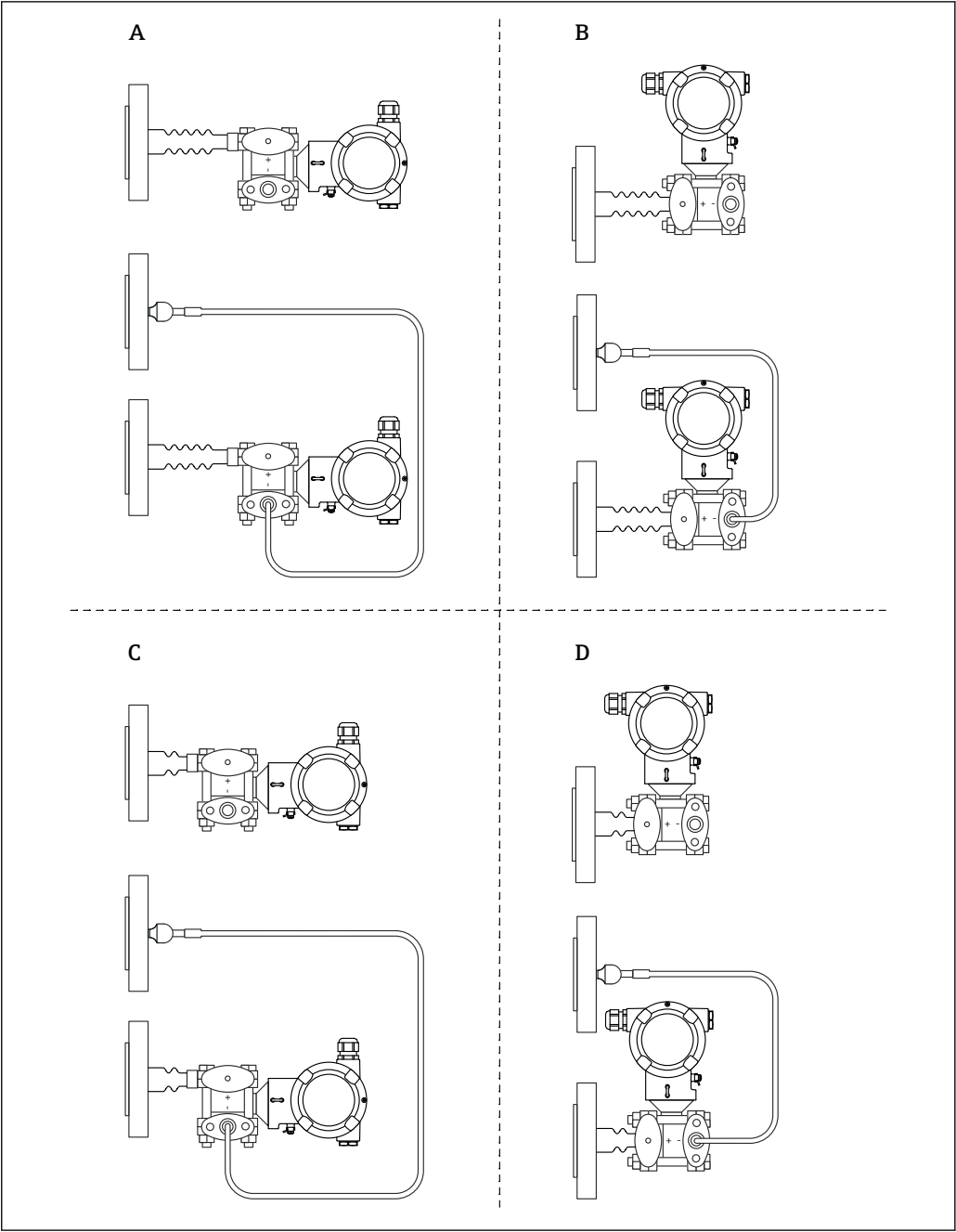
概覽：帶單側或雙側隔熱管隔膜密封系統的仪表
