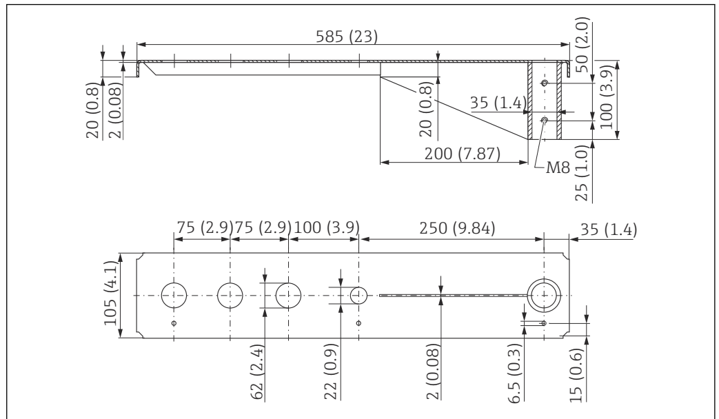
32 Dimensioni. Unità di misura mm (in)
