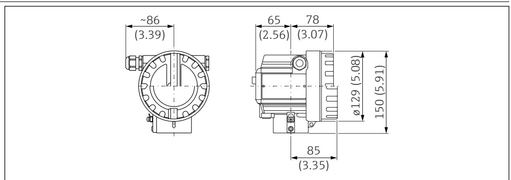
17 Dimensioni della custodia F12. Unità di misura mm (in)
