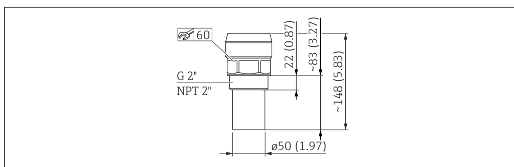
19 Dimensioni del sensore. Unità di misura mm (in)
