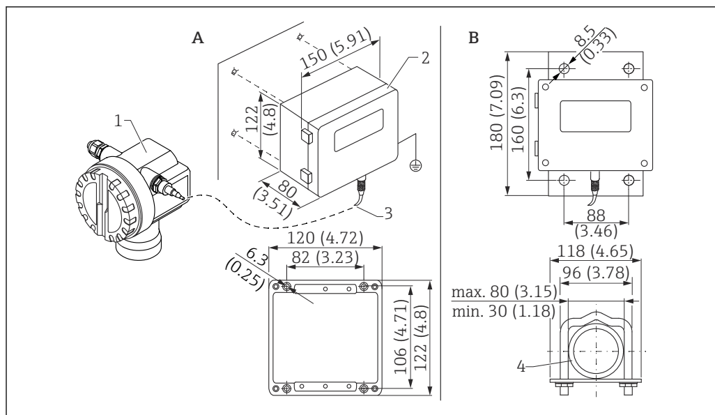
38 Indicador remoto. Unidad de medida mm (in)
