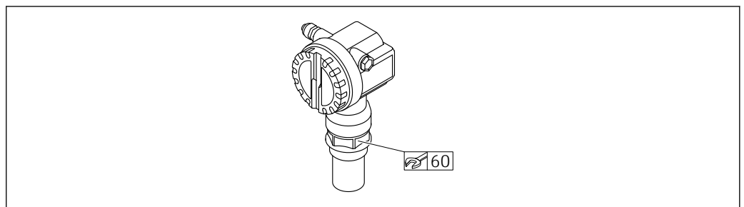
10 Montaje en reborde roscado, ancho entre caras AF60
