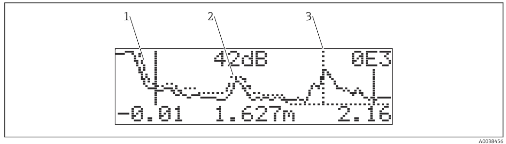
Fig. 29 Curva envolvente y mapeado
