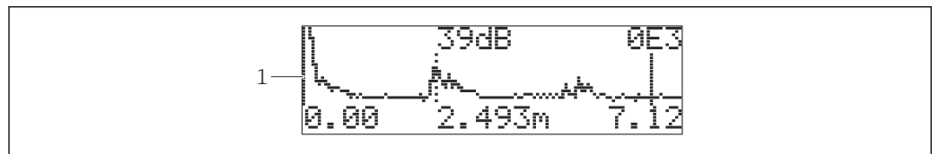
19 Visualización de la curva envolvente
