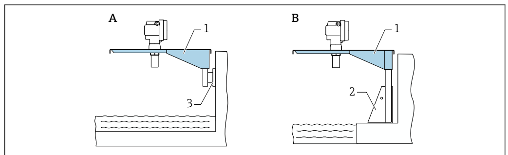
37 Soporte voladizo con soporte de montaje o placa de montaje en pared
