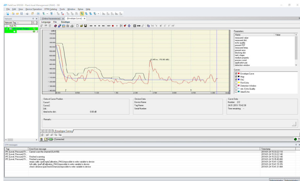
22 Análisis de la señal con curva envolvente, vista del software de configuración FieldCare
