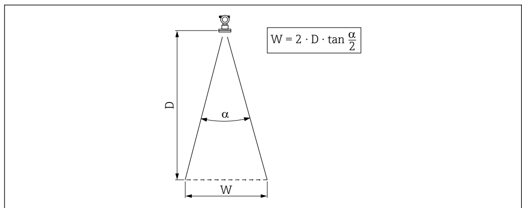
5 Relación entre el ángulo de abertura del haz \alpha , la distancia D y el diámetro del ancho del haz W
