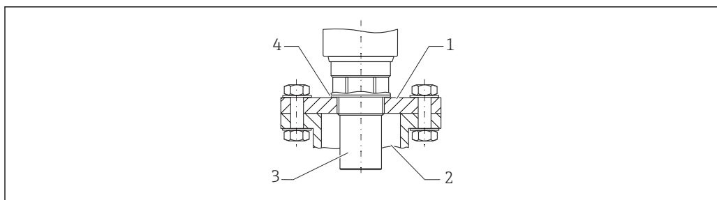
31 Brida de conexión roscada FAX50
