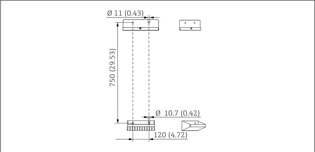
19 Dimensioni dell'unità di supporto Unità ingegneristica mm (in)
