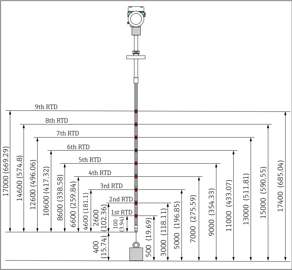
11 Position des éléments. Unité de mesure mm (in)
