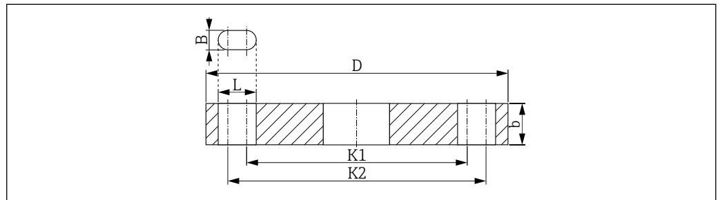
28 Abmessungen UNI Flansch FAX50
