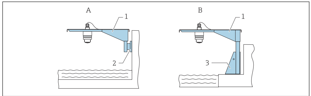
30 Montageart Sensor Prozessanschluss Rückseite
