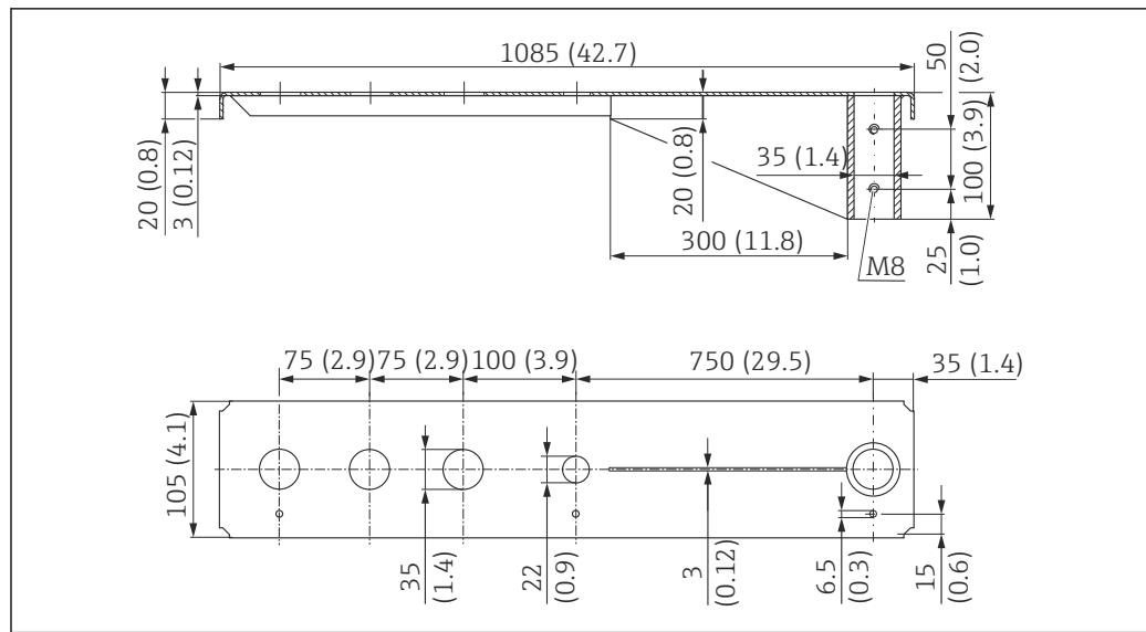
32 Abmessungen. Maßeinheit mm (in)
