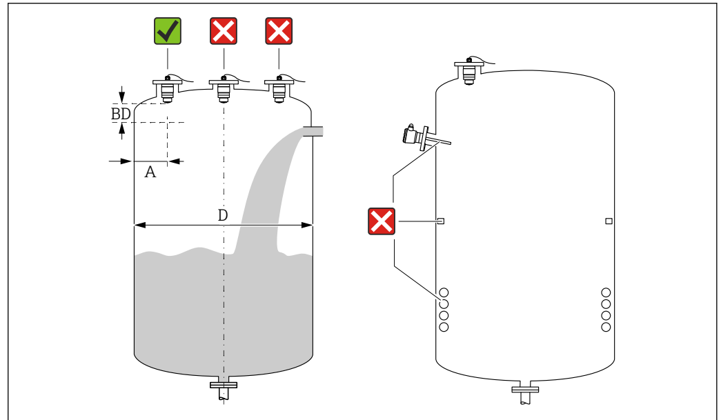
8 Behältereinbauposition
