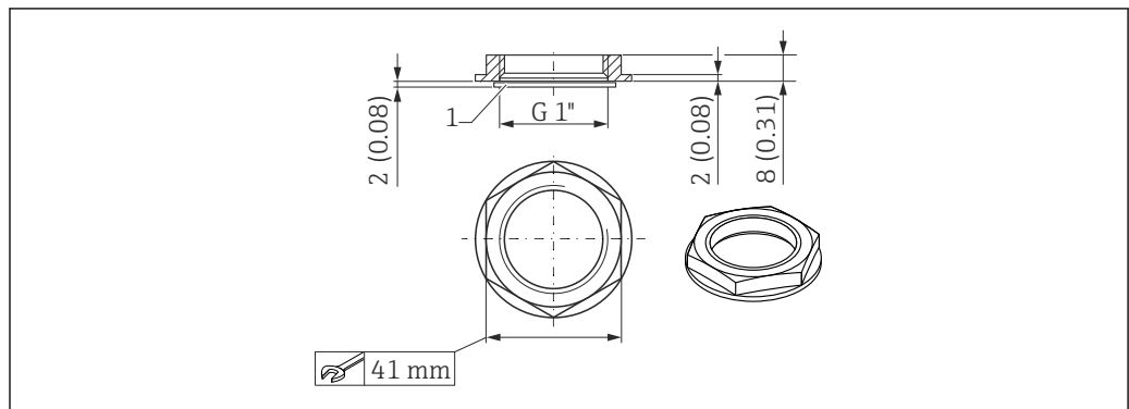
21 Abmessungen Gegenmutter Prozessanschluss Rückseite, Maßeinheit: mm (in)
