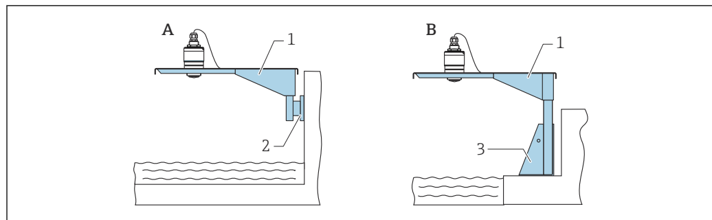
33 Montageart Sensor Prozessanschluss Vorderseite
