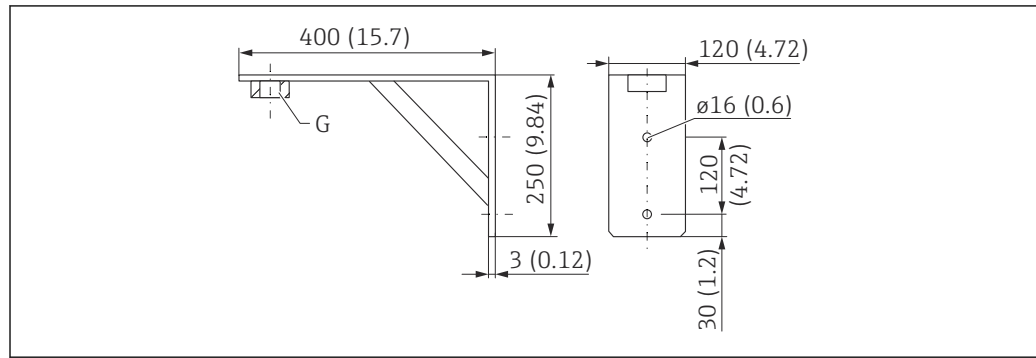
29 Abmessungen Montagewinkel. Maßeinheit mm (in)
