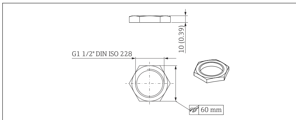
25 Abmessungen Befestigungsmutter, Maßeinheit: mm (in)
