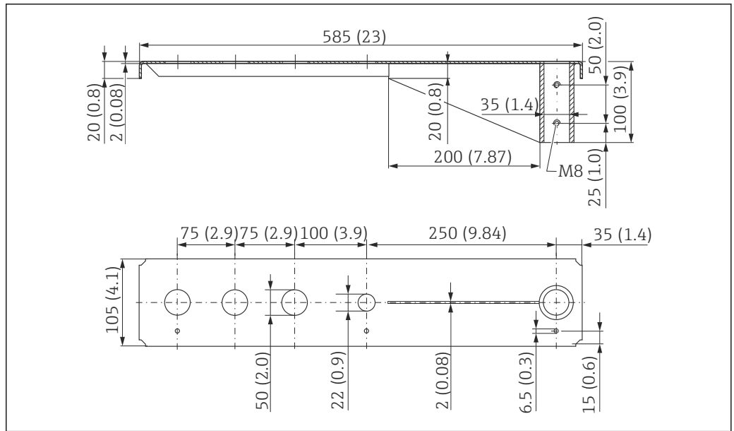
34 Abmessungen. Maßeinheit mm (in)
