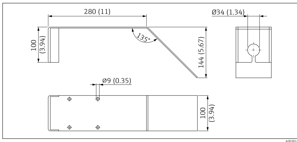
41 Abmessungen Horizontale Montagehalterung Abwasserschacht. Maßeinheit mm (in)
