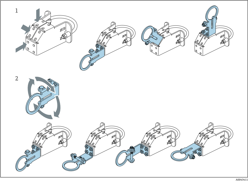
5 通过支架实现的调整选项 1 支架上的多个安装位置 2 通过转动支架
