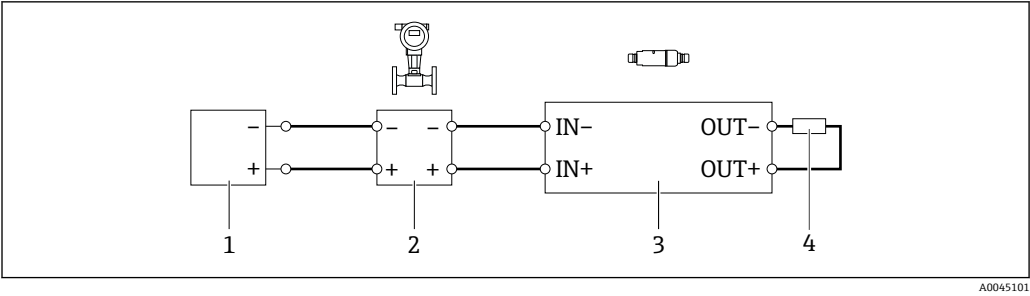
图 14 采用有源电流输出的四线制 HART 现场型设备的电气连接（可选接地未显示）- 接线端子 OUT 的电阻 1 四线制 HART 现场型设备供电电压（SELV、PELV 或 2 类） 2 采用有源 4...20 mA 输出的四线制 HART 现场型设备 3 电子插件 SWA50 4 250...500 Ω 的电阻，最小 250 mW（接线端子 OUT+和 OUT-之间）
