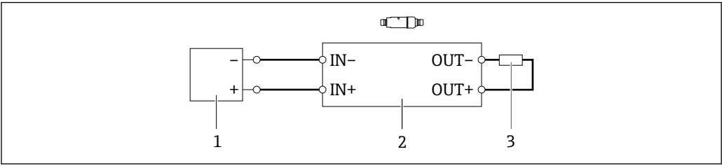
图 15 不带 HART 现场型设备的 FieldPort SWA50（可选接地未显示） 1 FieldPort SWA50 的供电电压，20...30 VDC（SELV、PELV 或 2 类） 2 电子插件 SWA50 3 1.5 kΩ 电阻，最小 0.5 W（接线端子 OUT+与 OUT-之间）
