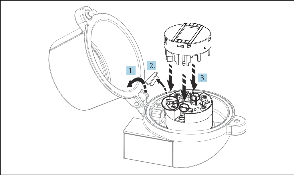
图 6 安装显示单元
