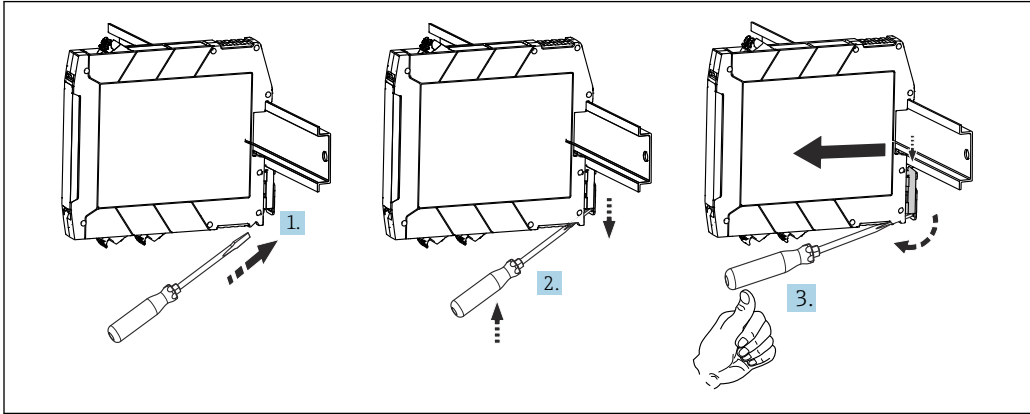
图 8 拆除 DIN 导轨盘装型变送器
