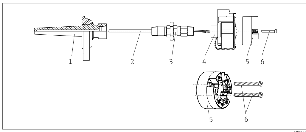
图 5 安装模块化变送器
