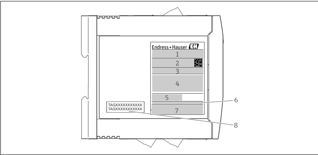
图 2 DIN 导轨型变送器的铭牌示例（图例为防爆型仪表的铭牌）
