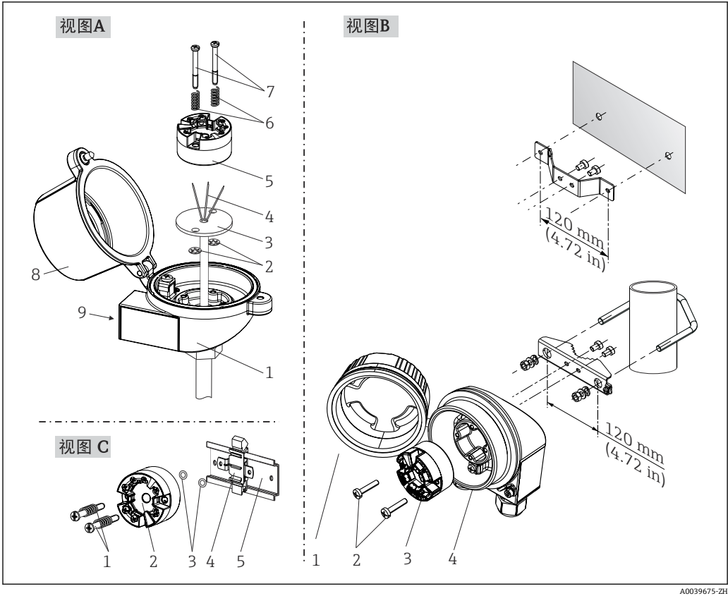
图 3 模块化变送器的安装示意图（三种安装方式）
