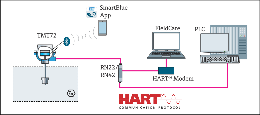
图 15 通过 HART®通信操作变送器
