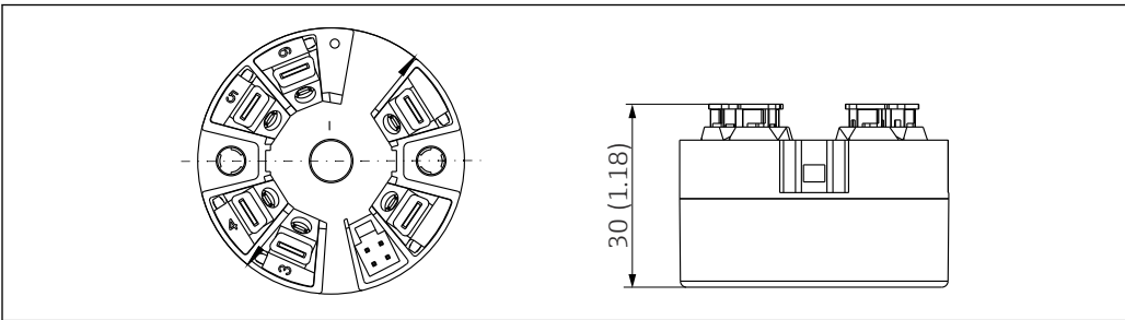
图 22 带直推式接线端子的仪表。除了外壳高度之外, 其他外形尺寸均与带螺纹式接线端子的仪表相同。
