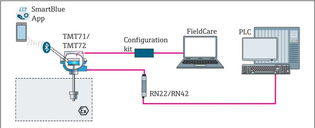
图 16 通过 CDI 接口操作变送器
