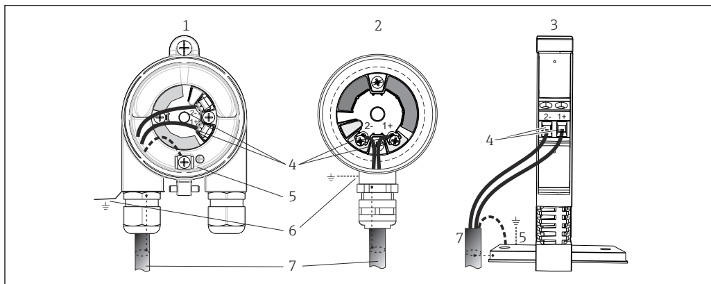
图 12 连接信号电缆和供电电缆
