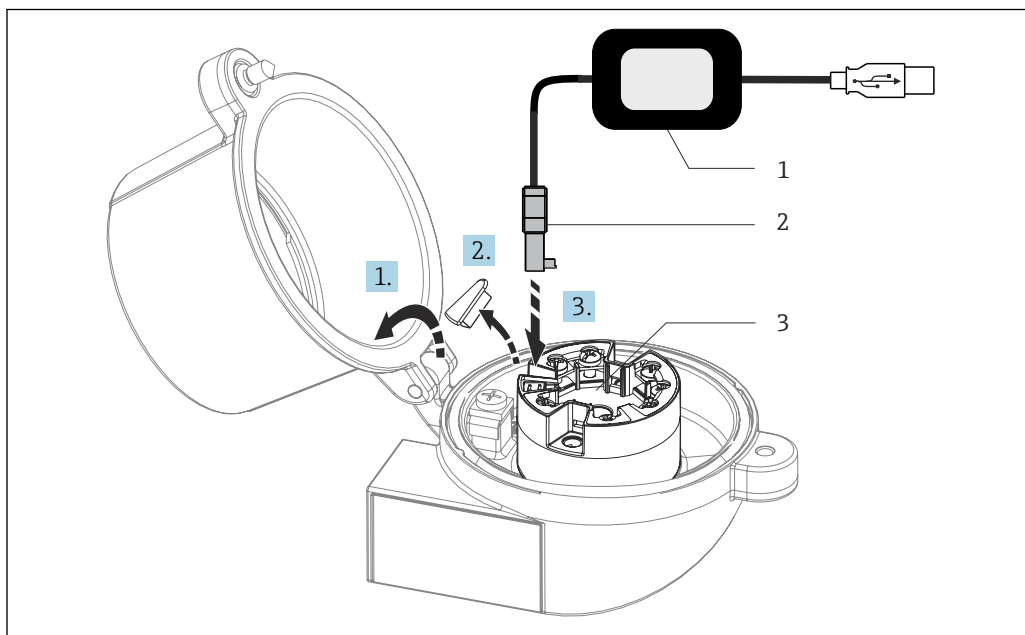
图 13 安装组态设置套件的 CDI 服务接口，通过 PC 机和组态设置软件进行模块化变送器的组态设置、可视化和维护操作
