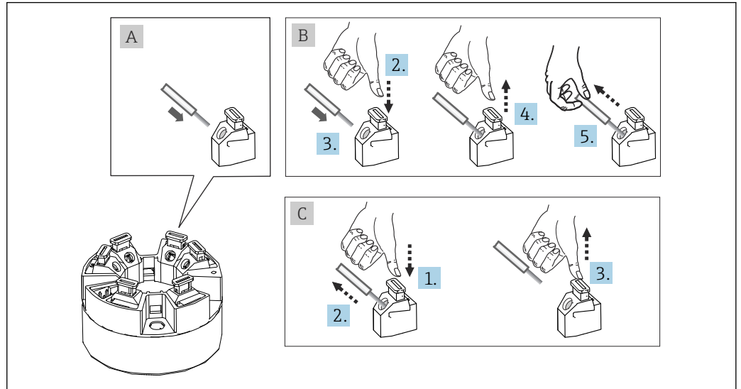
图 11 连接至直推式接线端子（以模块化变送器为例说明）
