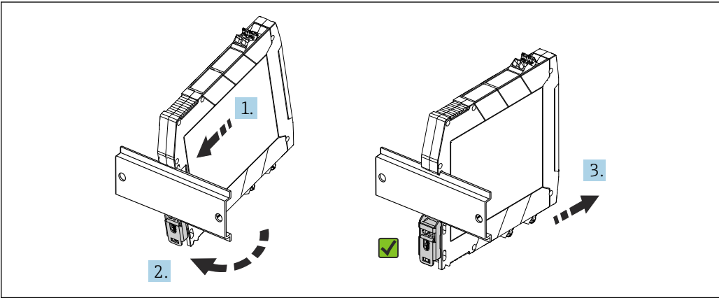
图 7 安装 DIN 导轨盘装型变送器
