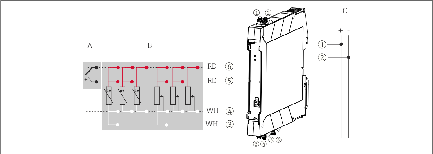
图 10 DIN 导轨型变送器的接线端子分配示意图 A 传感器输入，热电偶 (TC) 和电压 (mV) 信号 B 传感器输入，热电阻 (RTD) 和电阻 ( \Omega ) 信号，四线制、三线制和两线制连接 C 电源 4 ... 20 mA
