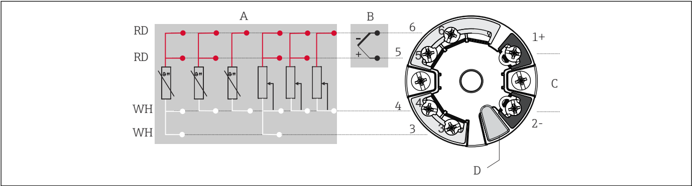
图 9 模块化变送器的接线端子分配 A 传感器输入，热电阻 (RTD) 和电阻 ( \Omega ) 信号，四线制、三线制和两线制连接 B 传感器输入，热电偶 (TC) 和电压 (mV) 信号 C 总线端连接器和电源 D 显示单元连接和 CDI 接口
