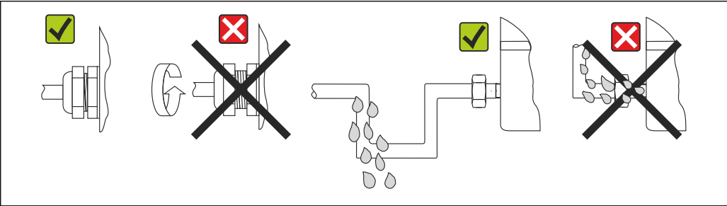
14 符合 IP67 防护等级的接线说明
