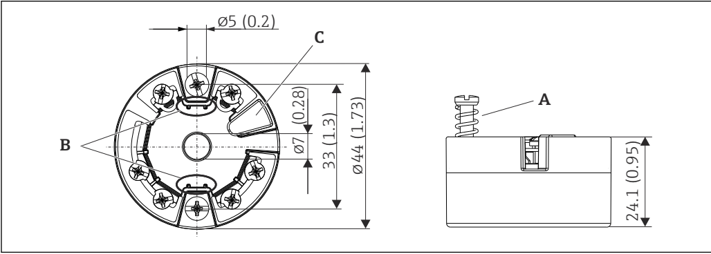
图 21 带螺纹式接线端子的仪表
