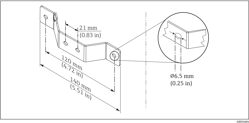
图 4 墙装架的外形尺寸（整套墙装套件可以作为附件订购）
