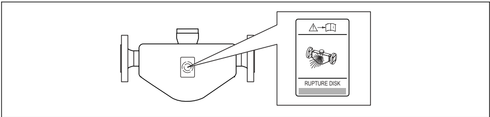
图 5 爆破片标签
