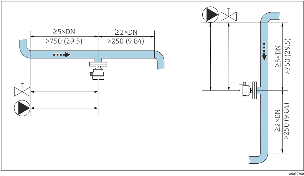
图 6 前直管段的安装。测量单位 mm (in)
