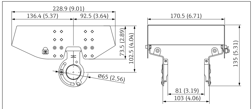
■ 18 防护罩，适用双腔室铝外壳。测量单位 mm (in)
