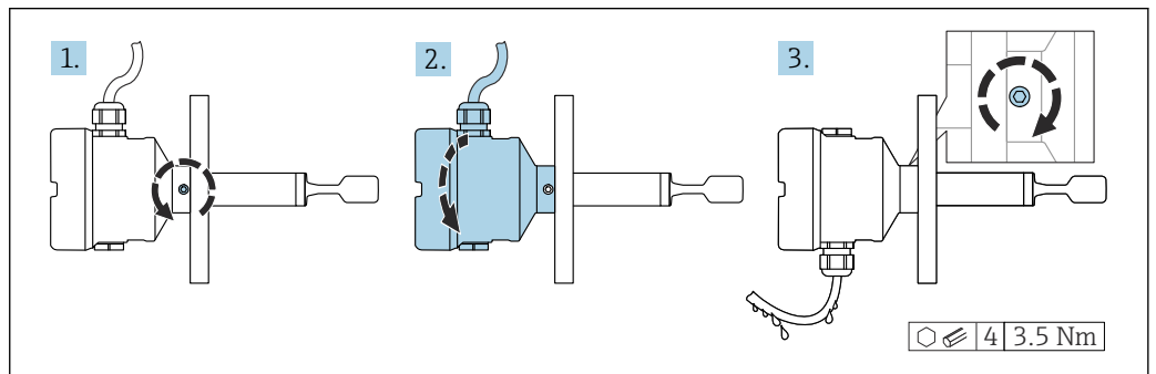
图 12 外壳带外部锁定螺丝和排水回路
