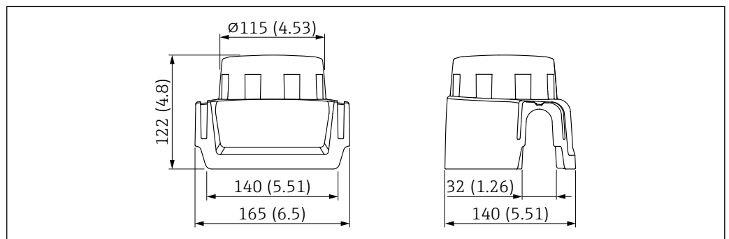
■ 19 防护罩，适用单腔室铝外壳或铸造 316L 外壳。测量单位 mm (in)
